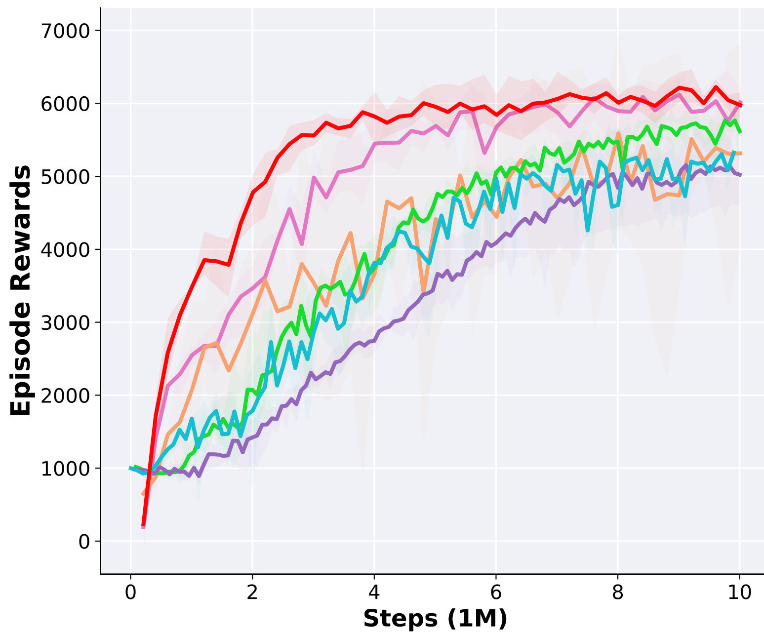
(d) Ant 2x4
