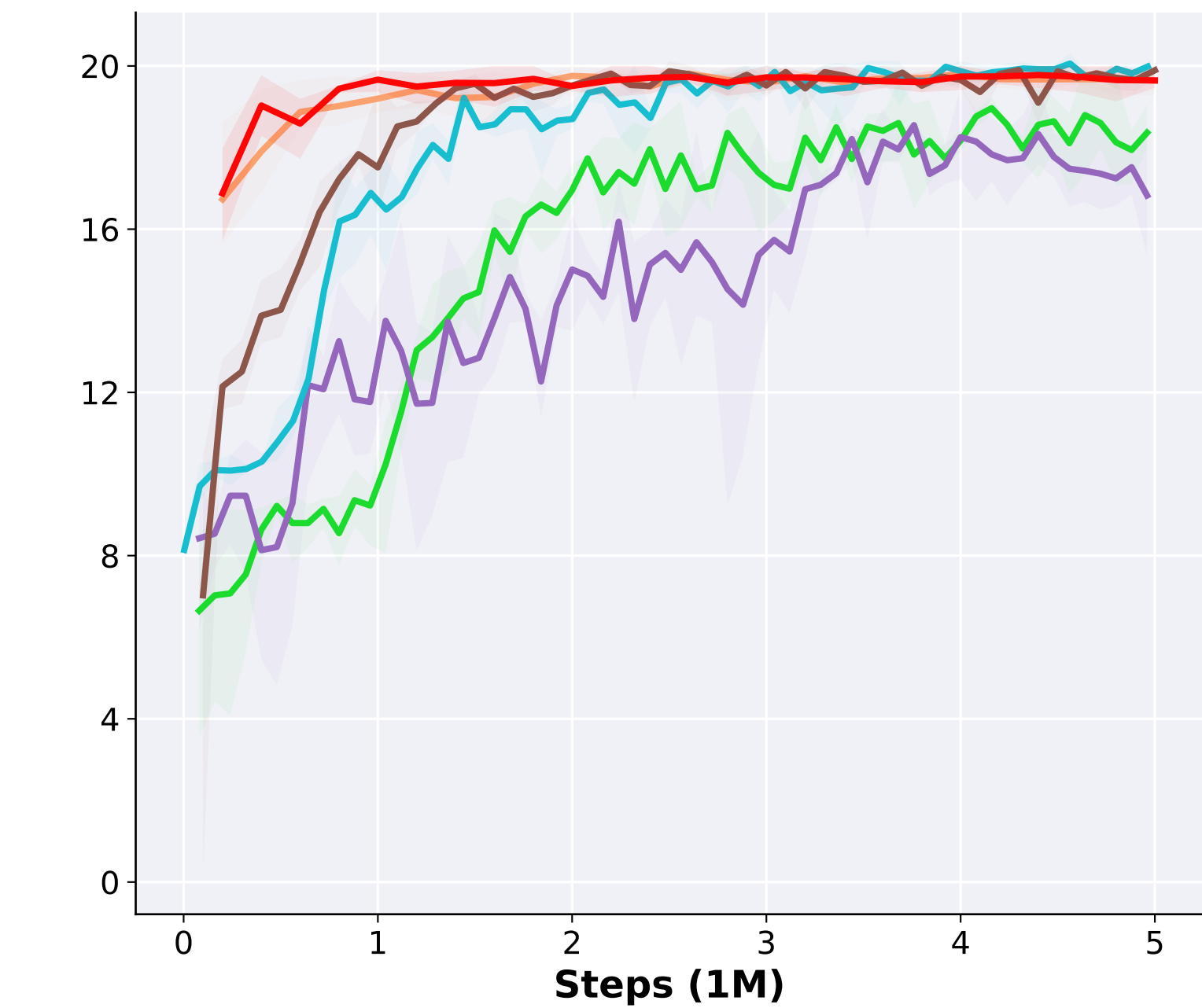
(f) 3s5z
