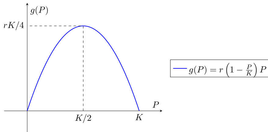
Figura 4.3: dP/dt para o modelo logístico.
