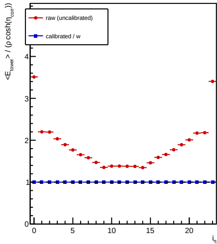
hcalin
