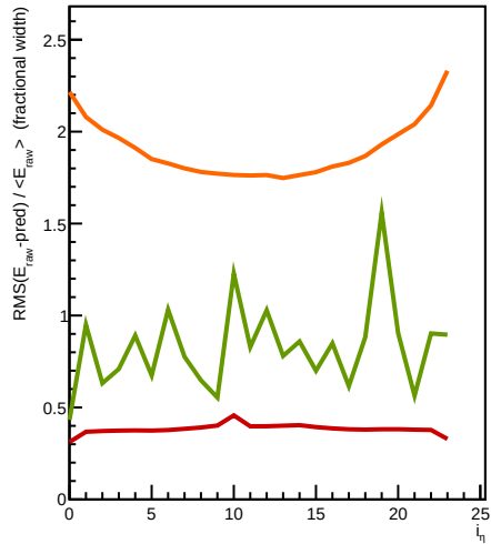
hcalin
