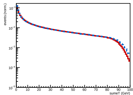
sumET HCALIN
