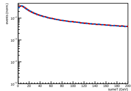
sumET CEMC
