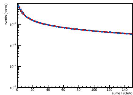
sumET HCALOUT
