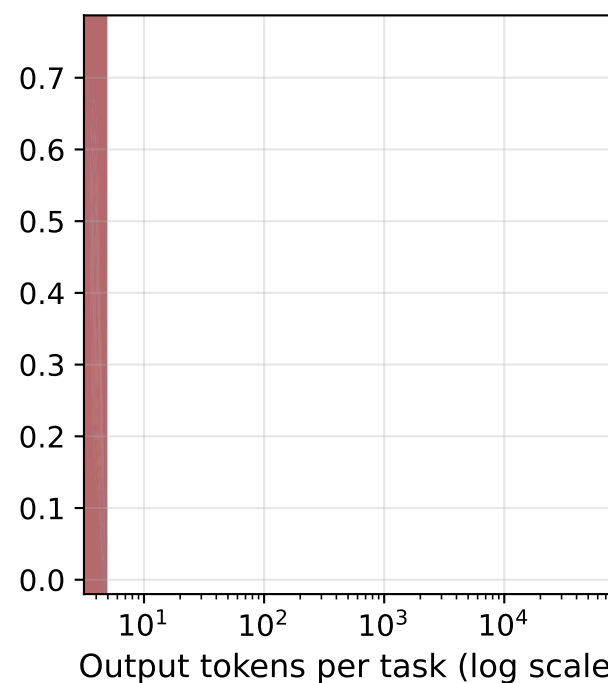
DirectLLM
