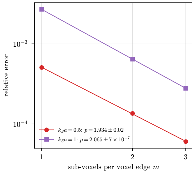
(d) voxelised sphere, fixed staircase
