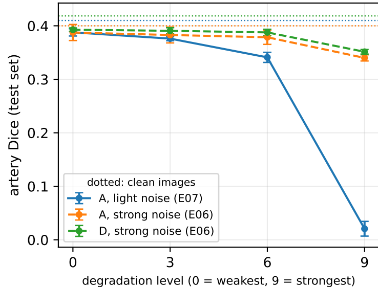
Poisson noise
