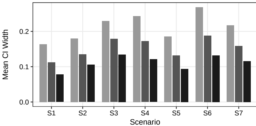
(C) CI Width
