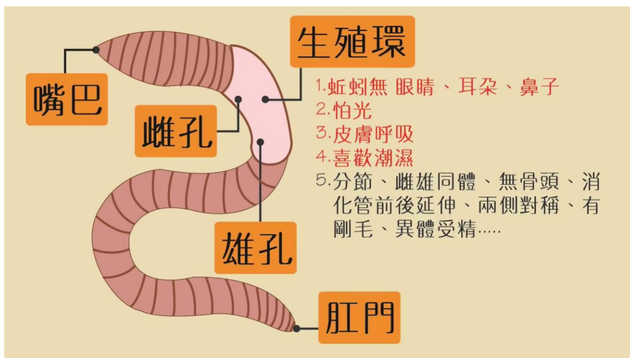
圖二：蚯蚓的構造
