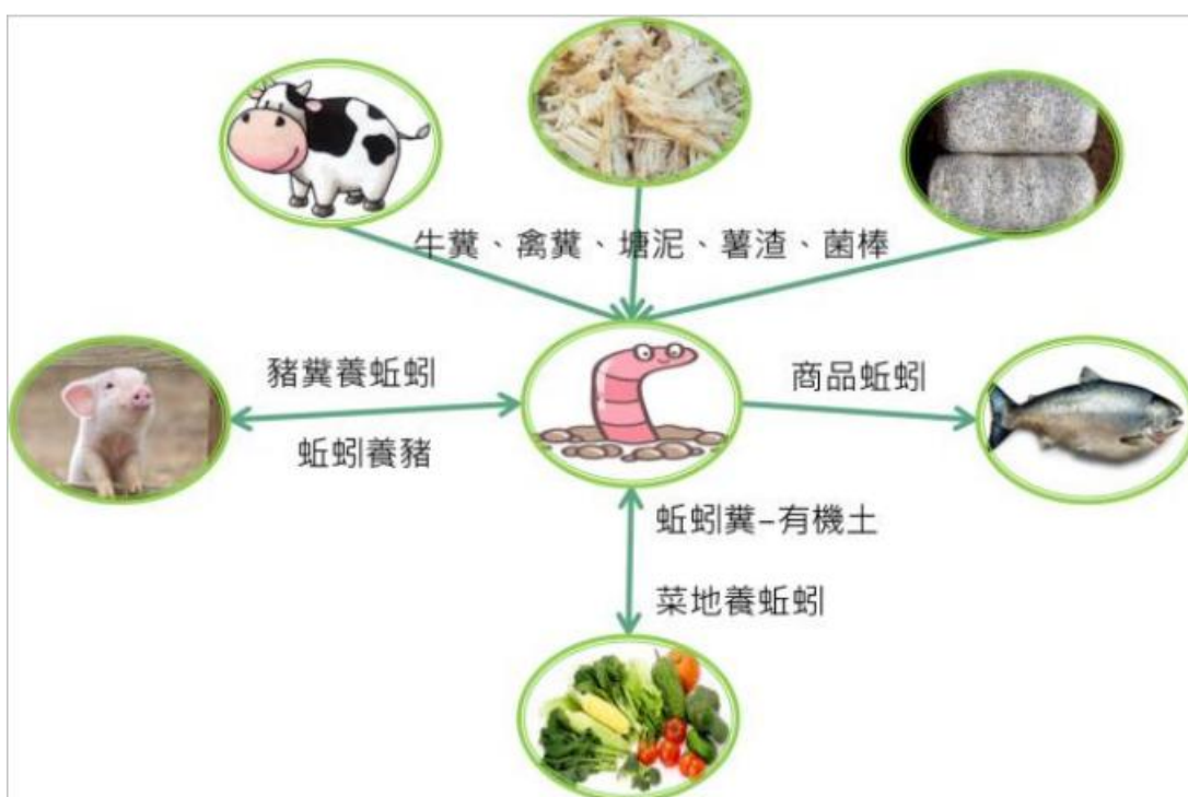
圖一：蚯蚓的循環友善環境概念
