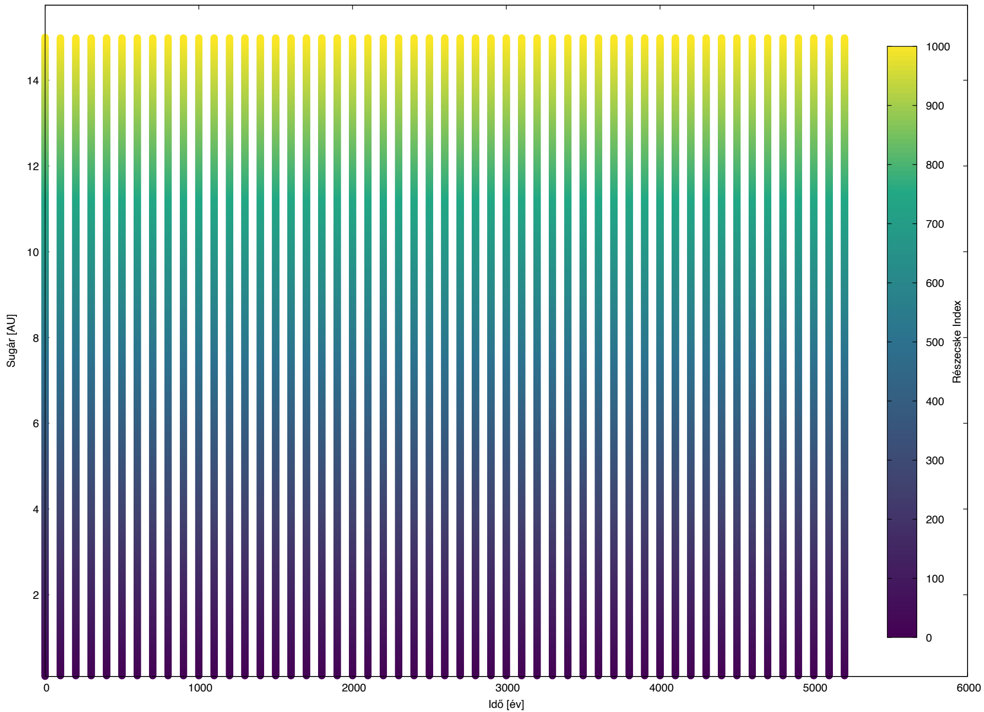
Porrészecskék sugarának evolúciója (Fixált Y-tengely: T=0 tartomány)
