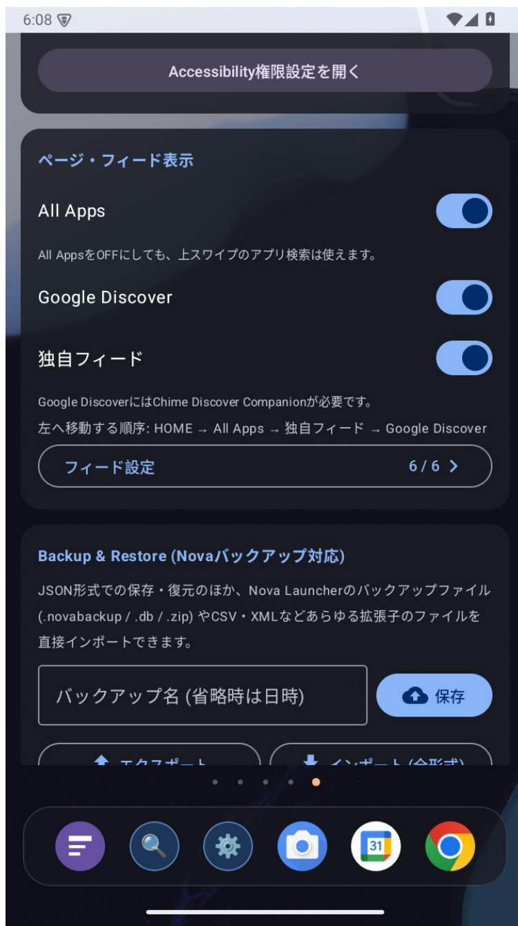
図20 : v1.3.8の「ページ・フィード表示」。Google Discover・独自フィード・All Appsを独立して切り替えます。
