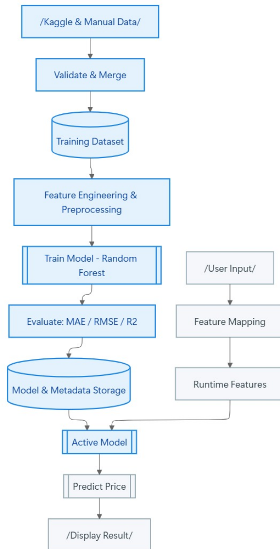
Hình 5.1: Sơ đồ luồng AI pipeline của hệ thống
