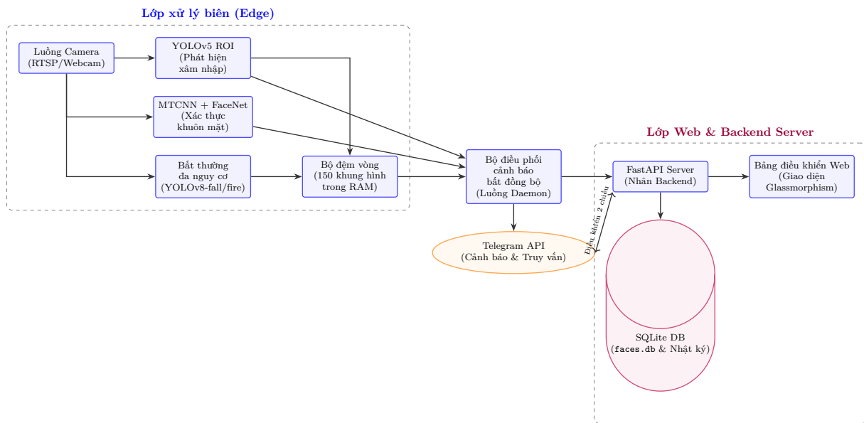
Hình 1: Sơ đồ kiến trúc và luồng dữ liệu hệ thống chi tiết
