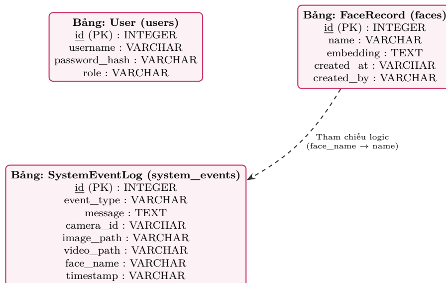
Hình 3: Sơ đồ thực thể liên kết (ER) của cơ sở dữ liệu
