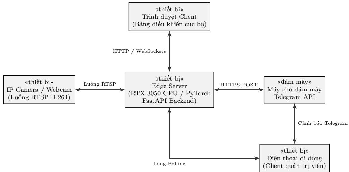
Hình 5: Sơ đồ triển khai phần cứng và phần mềm hệ thống
