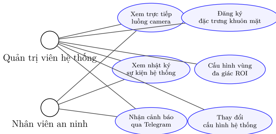
Hình 4: Mô hình Use Case cho hệ thống giám sát thông minh
