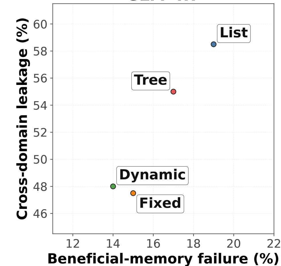
GLM-4.7
