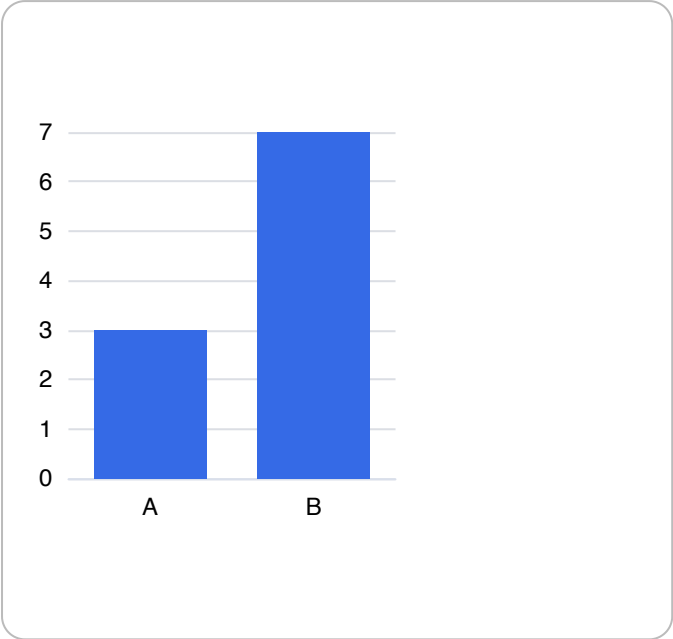
bar
