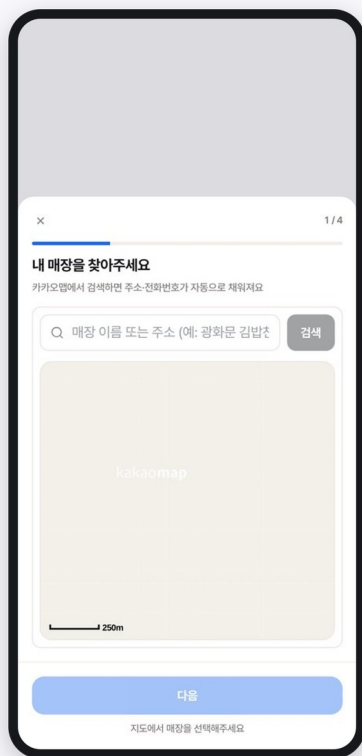
가게 찾기
