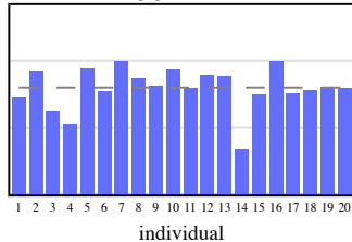
population 3
