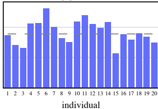
population 2
