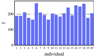
population 1
