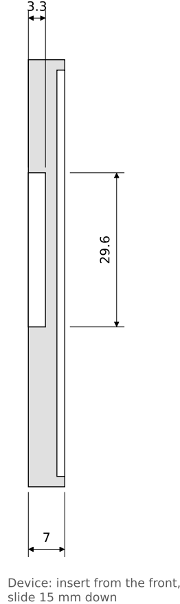
Section A-A (centre)
