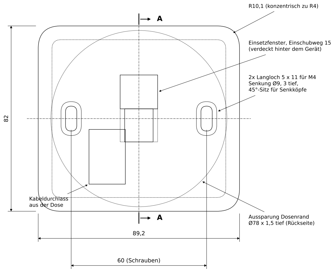
Wandplatte, Vorderansicht
