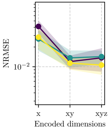
DV-QRC
