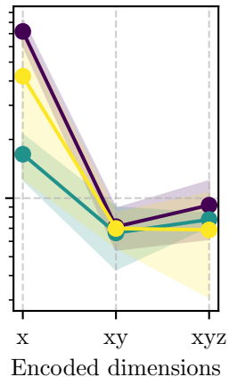
CV-QRC
