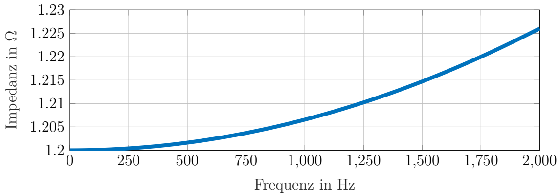
Abbildung 3.5: Frequenzabhängiger Impedanzverlauf einer der Spulen
