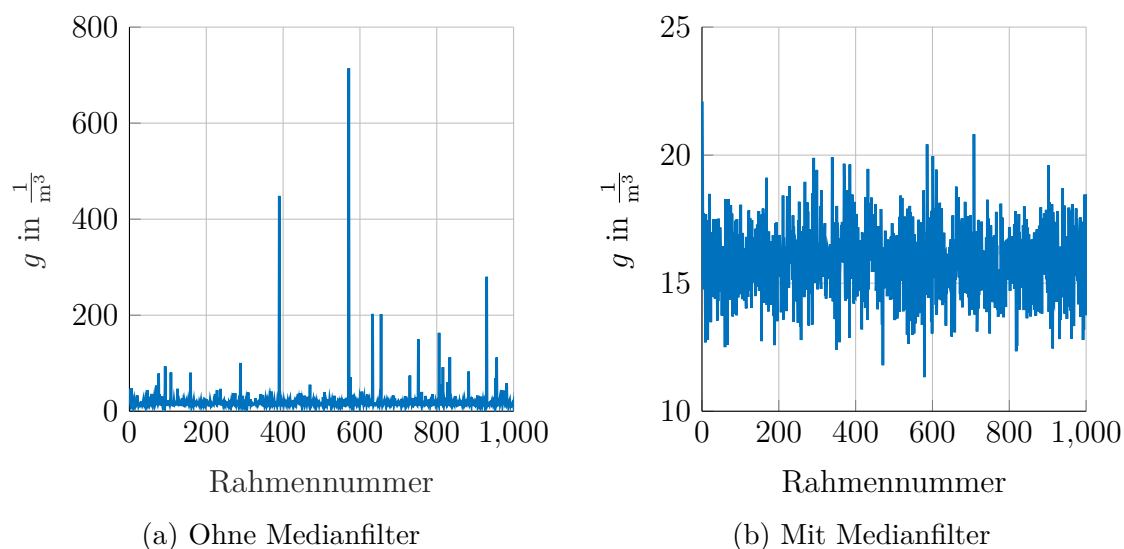
Abbildung 4.7: Auswertung des Distanzmerkmals anhand eines Laborsignals: In (a) ist der Verlauf des Distanzmerkmals ohne Medianfilter dargestellt, zum Vergleich dazu ist in (b) der Verlauf mit Medianfilter dargestellt. Die Rahmenlänge beträgt 512.
