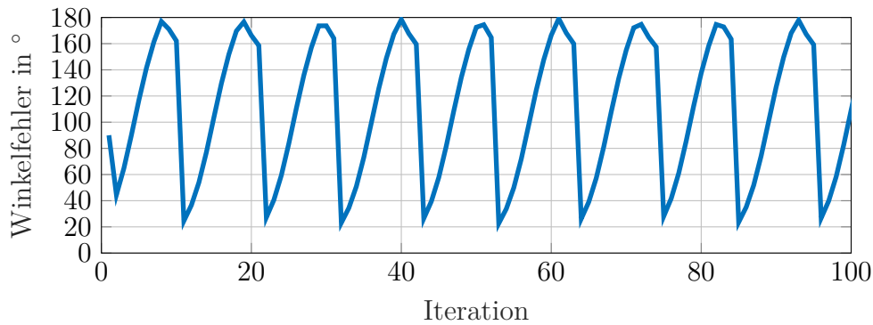
Abbildung 4.15: Winkelfehler für Q = 1 : Der Winkelfehler ist in Abhängigkeit der Iteration dargestellt.
