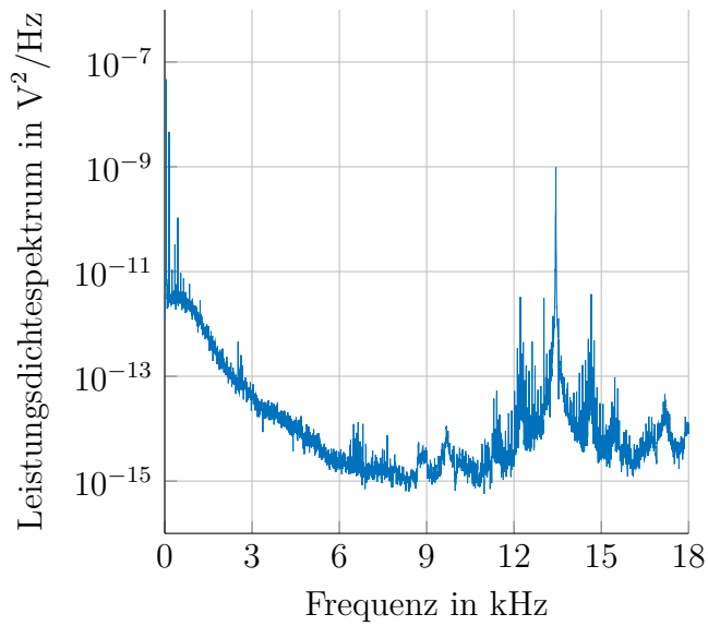
(a) Rauschspektrum
