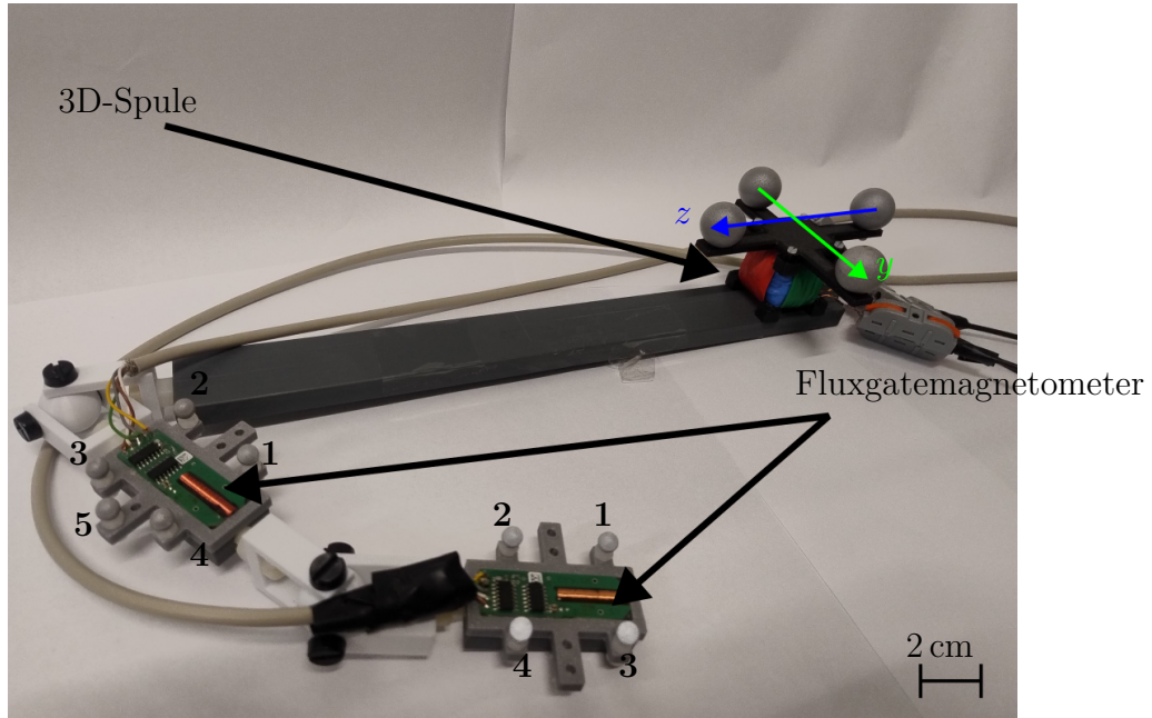
Abbildung 5.7: Demonstrator: Die Abbildung zeigt den Demonstrator, der für die Evaluierung verwendet wird. Die 3D-Spule und die kinematischen Elemente sind mit optischen Markern ausgerüstet.
