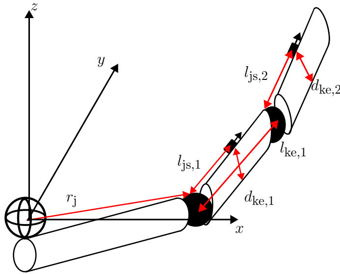
Abbildung 5.7: Kalibrierung der kinematischen Kette: Die Abbildung zeigt eine kinematische Kette bestehend aus drei Elementen. Die Roten Pfeile zeigen alle Größen die für den Algorithmus vor der Laufzeit bestimmt werden müssen.
