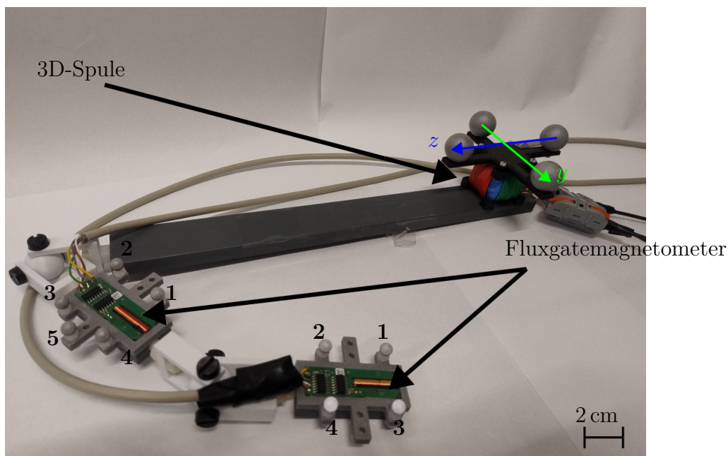
Abbildung 5.5: Demonstrator: Die Abbildung zeigt den Demonstrator, der für die Evaluierung verwendet wird. Die 3D-Spule und die kinematischen Elemente sind mit optischen Markern ausgerüstet.
