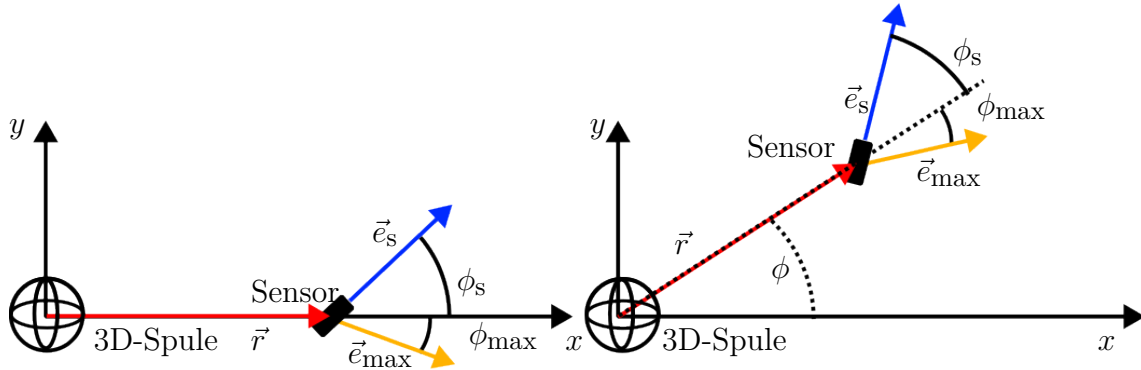
Abbildung 3.7: Die Beziehung aus Gleichung 3.40 ist unabhängig vom Winkel \phi . Außerdem wird die eindeutige Beziehung zwischen den drei Einheitsvektoren gezeigt. Auf der linken Seite ist der Sensor auf der x -Achse lokalisiert, wie in der Herleitung. Auf der rechten Seite ist der Aufbau gedreht. \phi_s und \phi_{\max} bleiben gleich, nur die Bezugsachse dreht sich mit.
