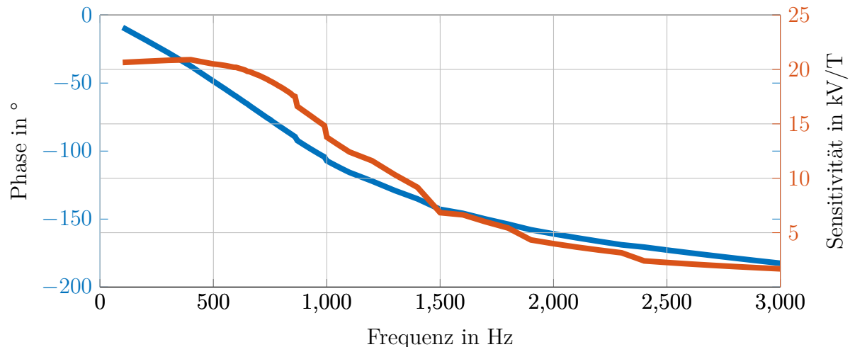
Abbildung 2.6: Verlauf von Sensitivität und Phase in Abhängigkeit der Frequenz
