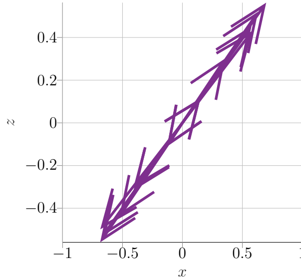
Abbildung 5.7: \vec{e}_{zc} aus einem der simulierten Rahmen: Für einen unbewegten Sensor ohne Rauschen liegen die Vektoren immer in einer Ebene, hier ist gut zu erkennen, dass dies für einen bewegten Sensor nicht gilt.
