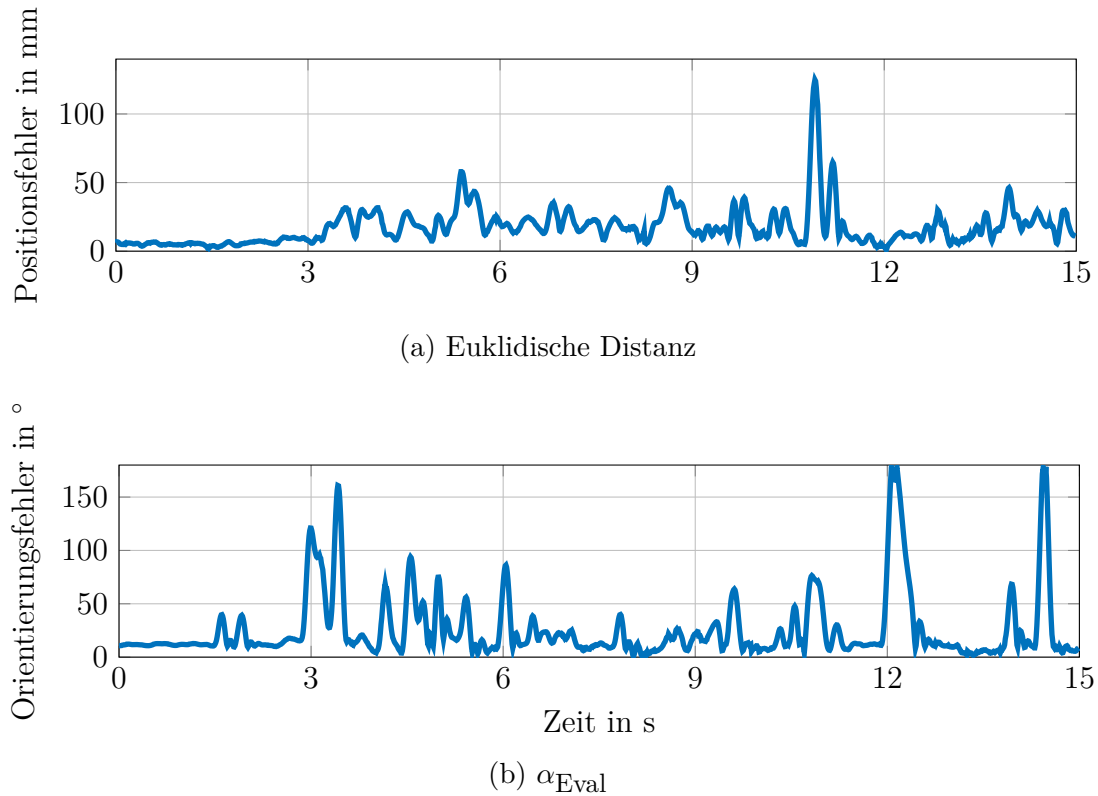
Abbildung 5.24: Fehler der dynamischen Messung über die Messsequenz
