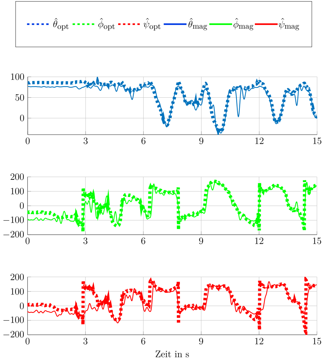
Abbildung 5.23: Ergebnis der dynamischen Evaluation der Orientierungsschätzung: Die optischen Schätzungen sind gestrichelt.
