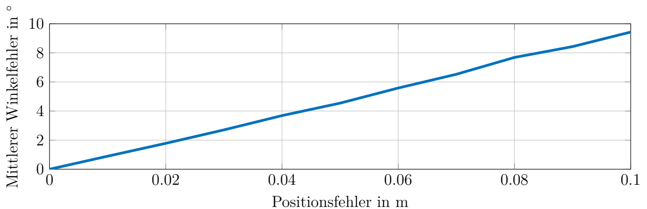
Abbildung 5.19: Mittelwert des Orientierungsfehlers in Abhängigkeit vom Positionsfehler
