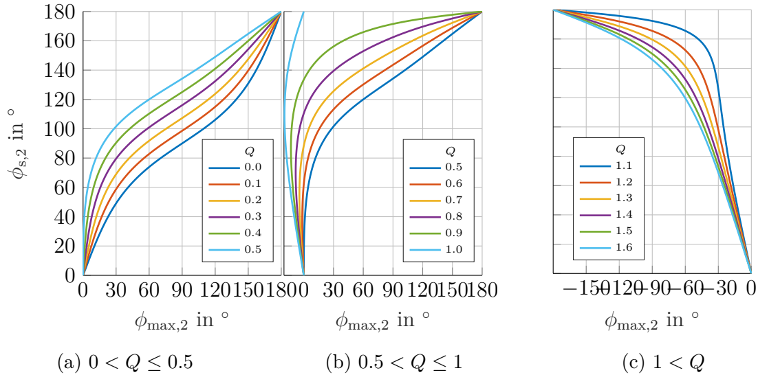
Abbildung 4.14: Funktionaler Winkelzusammenhang: In der Abbildung ist der Zusammenhang zwischen \phi_{s,2} und \phi_{m,2} für verschiedene Wertebereiche von Q . Die Abbildungen 4.14a und 4.14c zeigen eine eindeutige Zuordnung zwischen \phi_{s,2} und \phi_{m,2} . In diesem Bereich gibt es für jeden Eingangsvektor einen zugehörigen Ausgangsvektor. In Abbildung 4.14b ist der Zusammenhang für 0.5 < Q \leq 1 zu sehen. Hier sind teilweise einem Wert für \phi_{m,2} zwei unterschiedliche Werte für \phi_{s,2} zugeordnet.
