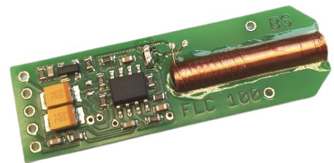
(b) Fluxgatemagnetometer FLC100 [23]
