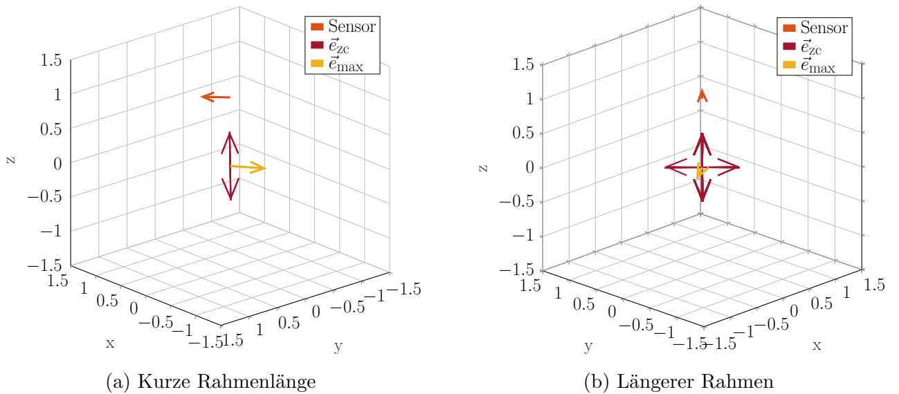
Abbildung 5.7: (a) zeigt die \vec{e}_{zc} s für eine Rahmenlänge 512, darin ist gut zu sehen, dass alles \vec{e}_{zc} = \pm \vec{e}_z sind. (b) zeigt dasselbe jedoch für eine Rahmenlänge von 4096. Dabei gibt es auch \vec{e}_{zc} s die nicht in z -Richtung polarisiert sind.
