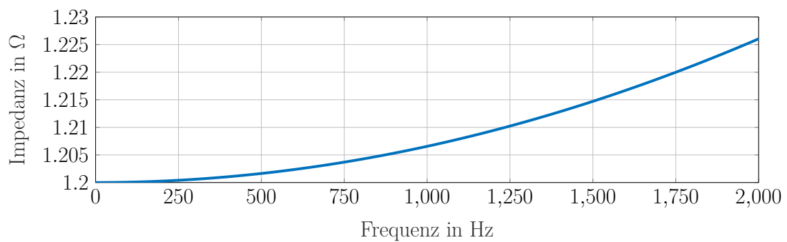
Abbildung 3.5: Frequenzabhängiger Impedanzverlauf der 3D-Spule
