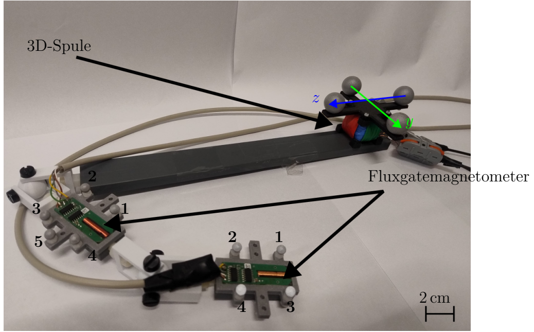
Abbildung 5.1: Demonstrator: Die Abbildung zeigt den Demonstrator, der für die Evaluierung verwendet wird. Die 3D-Spule und die kinematischen Elemente sind mit optischen Markern ausgerüstet.
