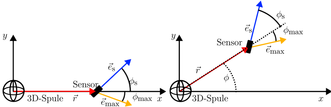
Abbildung 3.7: Die Beziehung aus Gleichung 3.40 ist unabhängig vom Winkel \phi . Außerdem wird die eindeutige Beziehung zwischen den 3 Einheitsvektoren \vec{e}_s , \vec{e}_{\max} , und \vec{e}_r gezeigt. Auf der linken Seite ist der Sensor auf der x -Achse lokalisiert, wie in der Herleitung. Auf der rechten Seite ist das Ganze Setup gedreht. \phi_s und \phi_{\max} bleiben gleich, nur die Bezugsachse dreht sich mit.
