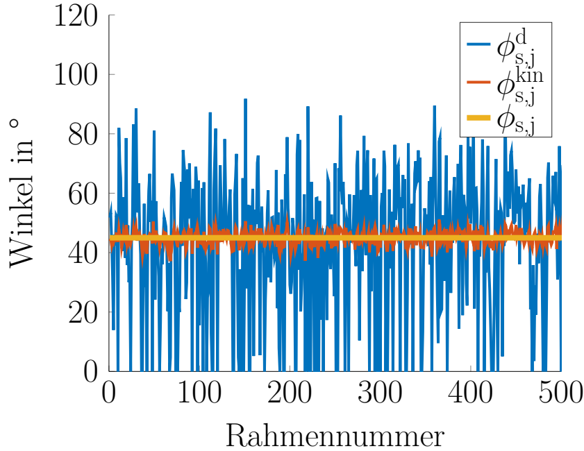
Abbildung 4.23: Vergleich der unterschiedlichen Berechnungsmethoden für \phi_{s,2} : Gelb zeigt den wahren Wert, Orange den aus dem vorgestellten Algorithmus und Blau den aus der Distanz bestimmten Wert.
