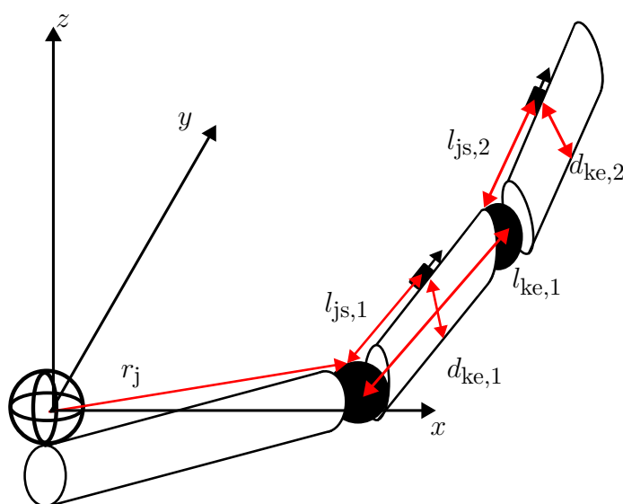
Abbildung 5.10: Kalibrierung der kinematischen Kette: Die Abbildung zeigt eine kinematische Kette bestehend aus drei Elementen. Die Roten Pfeile zeigen alle Größen die für den Algorithmus vor der Laufzeit bestimmt werden müssen.
