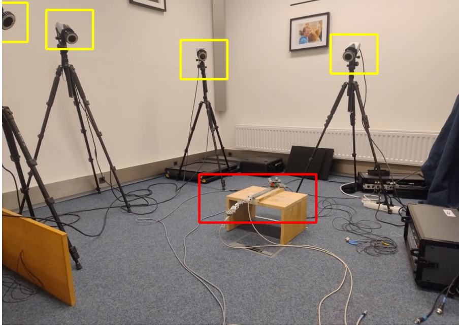
Abbildung 5.8: Evaluierungsaufbau: Das Foto zeigt den Demonstrator in der Mitte (rot) und im Außenbereich die Kameras (gelb).
