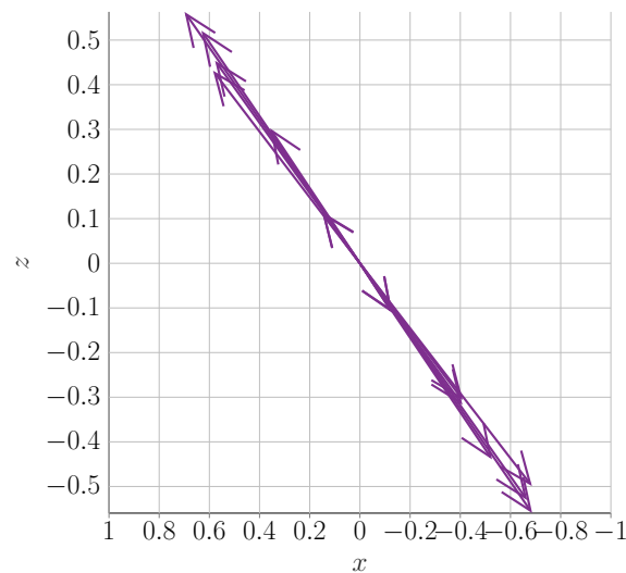
Abbildung 5.8: Nulldurchgangsvektoren die aus einem der simulierten Rahmen extrahiert wurden. Für einen unbewegten Sensor ohne Rauschen liegen die Vektoren immer in einer Ebene, hier ist gut zu erkennen, dass dies für einen bewegten Sensor nicht gilt.
