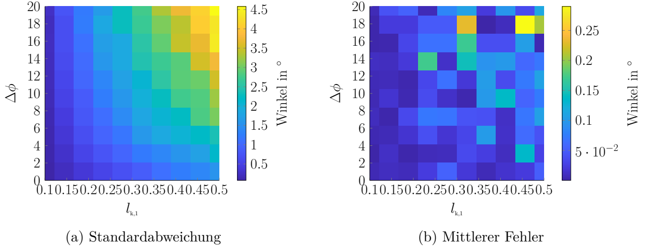
Abbildung 5.5: Auf der linken Seite ist die Standardabweichung der Orientierung in Abhängigkeit des falsch angenommenen Winkels und der Länge des mittleren Elements. In der rechten Abbildung sind die Fehler des über 100 Schätzungen gemittelten Werts dargestellt.
