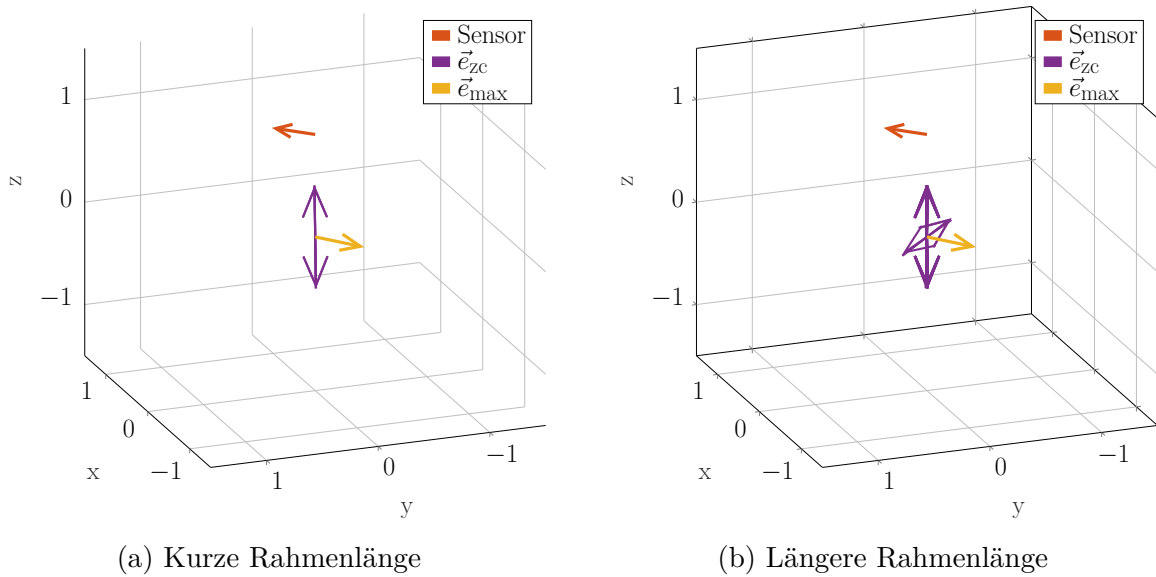
Abbildung 5.7: (a) zeigt die \vec{e}_{zc} s für eine Rahmenlänge 512. (b) zeigt dasselbe für eine Rahmenlänge von 4096.
