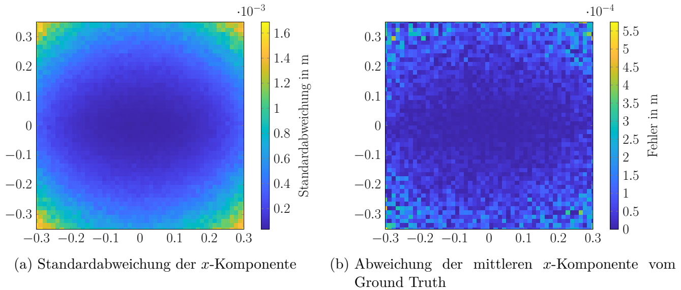
Abbildung 5.18: Ergebnisse der Simulation zur Überprüfung der Robustheit der Positionsschätzung gegen weißes Rauschen
