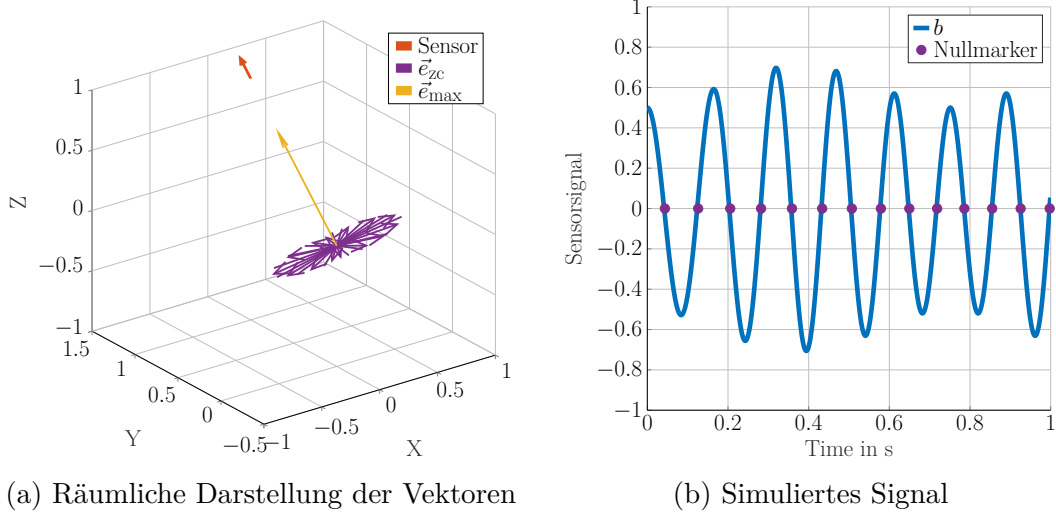
Abbildung 4.6: Die linke Abbildung zeigt beispielhaft einen MV im Ursprung (gelb), die Position und Orientierung (orange) des Sensors und die entsprechende Ebene der Nulldurchgangsebene (lila). Auf der rechten Seite ist das entsprechende Sensorsignal als Funktion der Zeit dargestellt. Die Zeiten, in denen ein Nulldurchgang erreicht wird, sind mit einem lila Punkt markiert. Die Simulation arbeitet mit einer Quelle, die mit N_\omega = \omega_\theta/\omega_\phi = 10 angesteuert wird. Die absoluten Werte/Längen sind nicht relevant, da zum einen das relative Verhältnis zwischen den Vektoren und zum anderen die Nulldurchgänge von Interesse sind.
