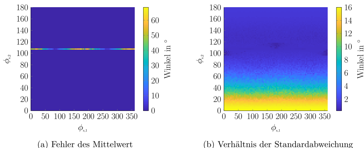
Abbildung 5.3: Die linke Abbildung zeigt den Fehler der Orientierung, nach einer Mittelung von 100 Schätzungen. Die rechte Seite zeigt das Verhältnis zwischen der Standardabweichung des MV und der Standardabweichung der Orientierung.
