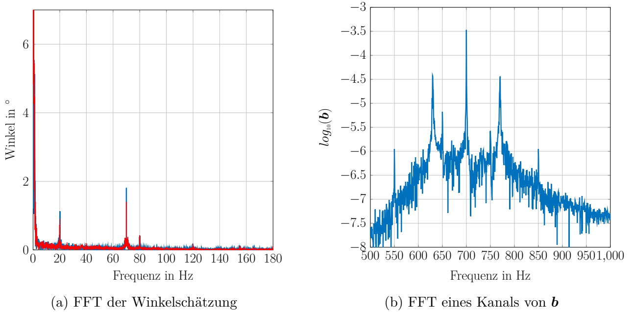
Abbildung 5.16: Frequenzanalyse der Winkelschätzung und der magnetischen Eingangssignale, es ist jeweils das Signal des ersten Elements dargestellt.
