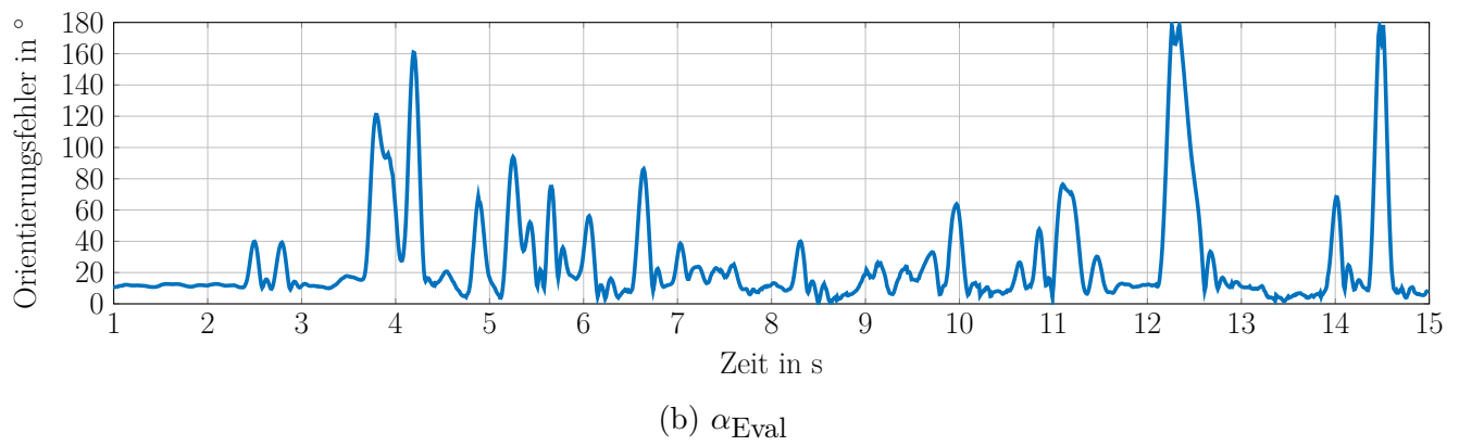
Abbildung 5.24: Fehler der dynamischen Messung über die Messsequenz
