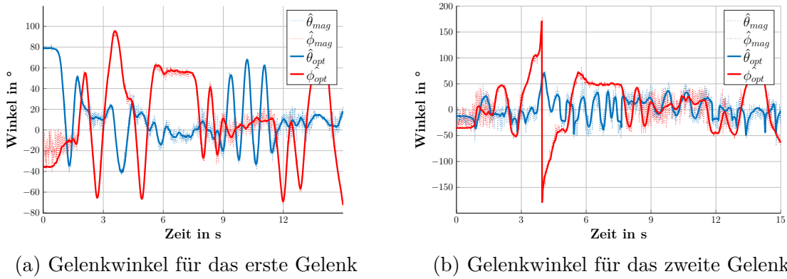
Abbildung 5.13: Die Abbildung zeigt die beiden Gelenkwinkel für das erste(a) und zweite Gelenk(b). Dabei sind die Schätzungen der magnetischen Lokalisierung ohne Nachverarbeitung(gestrichelt), sowie die optischen Schätzungen über der Zeit aufgetragen.
