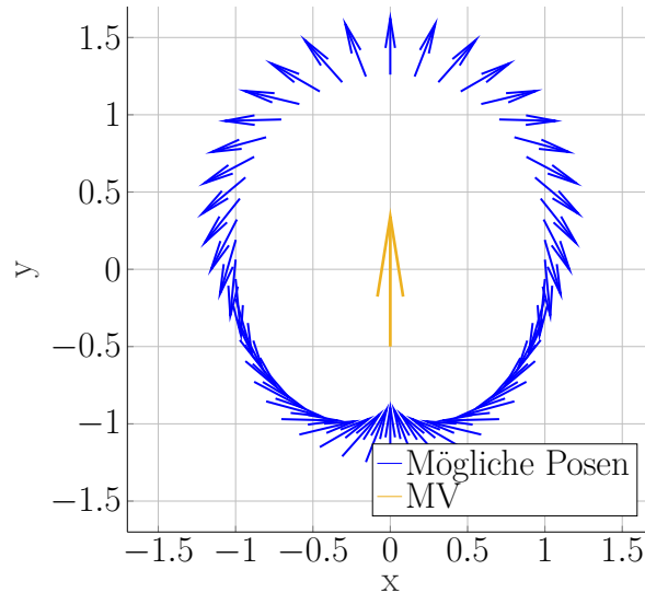
Abbildung 3.8: Potentielle Posen der Sensoren: In der Mitte ist ein MV in y -Richtung polarisiert. Die Blauen Vektoren zeigen potentielle Posen, Positionen mit den zugehörigen Orientierungen. Der Anfang der Pfeile definiert die Position und die Richtung des Pfeils die zugehörige Orientierung.
