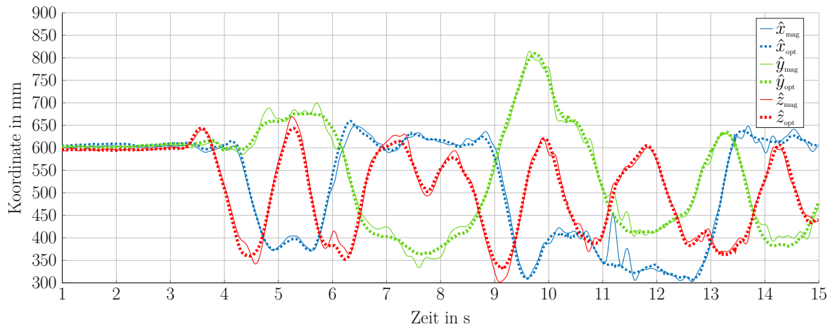
Abbildung 5.22: Ergebnis der dynamischen Evaluierung der Positionsschätzung: Es sind die drei Positionskomponenten dargestellt. Die magnetischen Schätzungen sind in durchgezogenen Linien und die optischen in gestrichelten Linien dargestellt.
