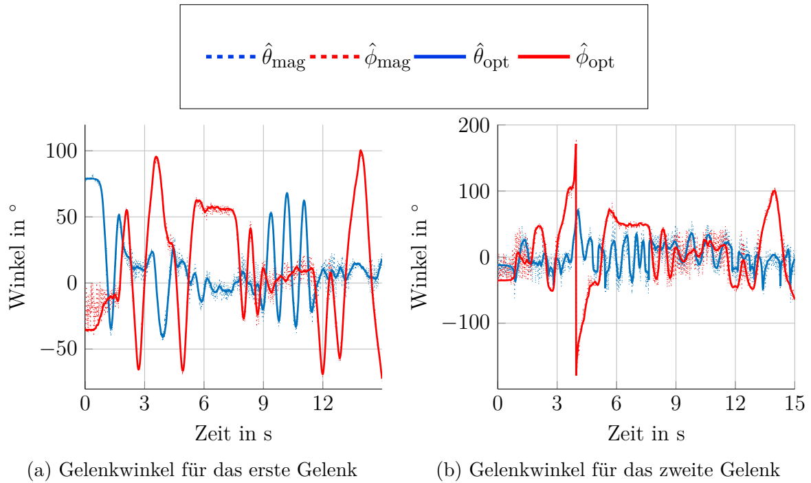
Abbildung 5.12: Die Abbildung zeigt die beiden Gelenkwinkel für das erste (a) und zweite Gelenk (b). Dabei sind die Schätzungen der magnetischen Lokalisierung ohne Nachverarbeitung (gepunktet), sowie die optischen Schätzungen über der Zeit aufgetragen.
