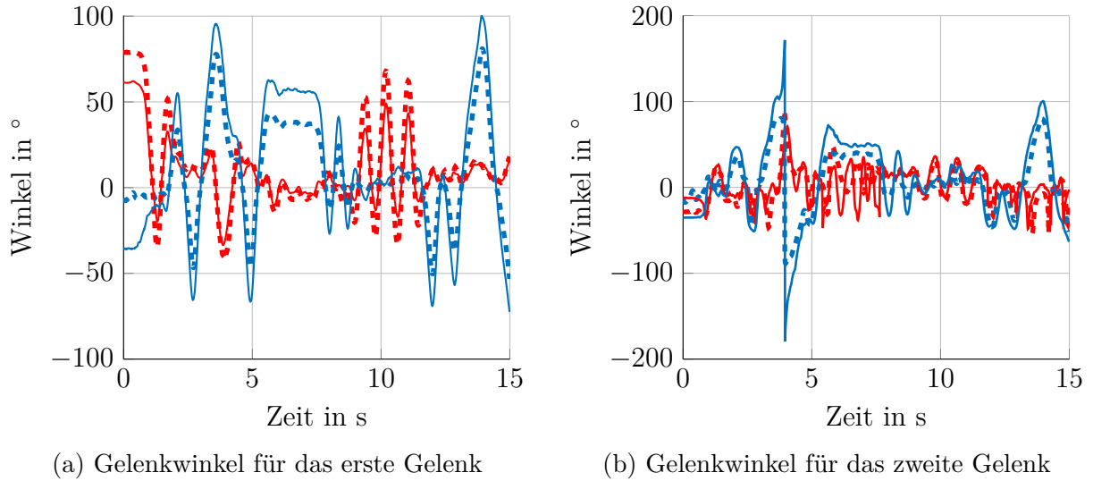
Abbildung 5.15: Ergebnis der Schätzung für die Verwendung eines LookUpTable
