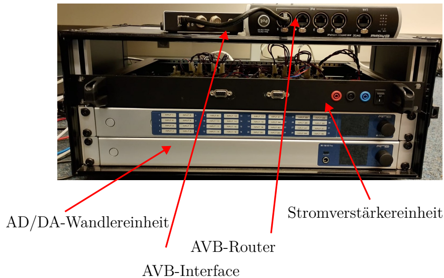
Abbildung 5.1: Die Abbildung zeigt die verwendete Hardware bestehend aus einem Labornetzteil, einer AD/DA-Wandlereinheit, einer Stromverstärkereinheit und einen AVB-Router mit Interface zum Auswertecomputer.
