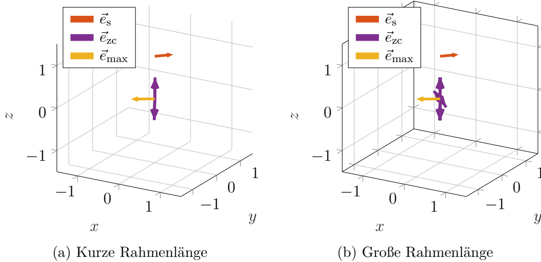
Abbildung 5.6: (a) zeigt die \vec{e}_{zc} für eine Rahmenlänge 512, (b) für eine Rahmenlänge von 4096.
