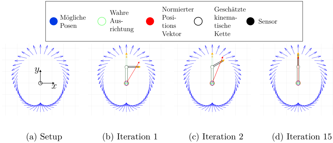
Abbildung 4.11: Beispielhafter iterativer Prozess: Die Abbildung zeigt die Iterationen für einen einfachen Aufbau. Die Unterabbildung (a) zeigt das Koordinatensystem. Der Ursprung dieses Aufbaus befindet sich am ersten kinematischen Kettenelement, wo sich auch die Quelle befindet. In den folgenden Unterabbildungen wurde das Koordinatensystem weggelassen. Die blauen Vektoren stellen die möglichen Posen für den detektierten MV dar. Die hellgrüne Konstruktion zeigt die wahre Ausrichtung der kinematischen Kette. Der rote Vektor ist ein normalisierter Positionsvektor des Sensors, der auf die potentielle Pose in dieser Richtung zeigt. Der Sensor ist am zweiten Element angebracht. Er wird durch einen orangenen gefüllten Kreis mit einem Vektor in die sensitive Richtung dargestellt. Unterabbildung (b) beginnt mit einer Elementausrichtung in x -Richtung. Für einige Iterationen sind die kinematische Kette und der zugehörige Positionsvektor dargestellt. Nach 15 Iterationen (Unterabbildung (d)) stimmt die Sensorpose mit einer potentiellen Pose überein und der Algorithmus konvergiert.
