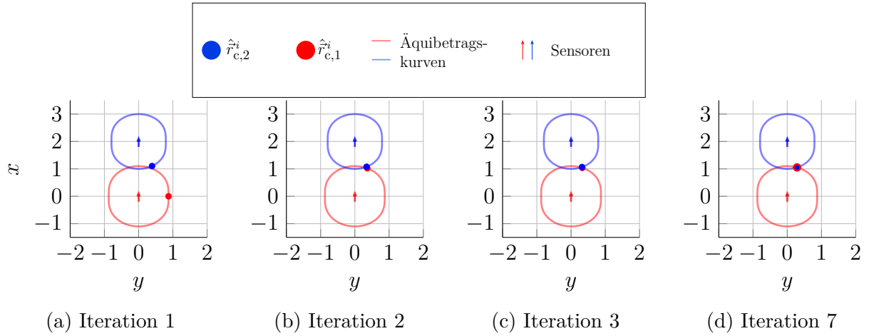
Abbildung 4.18: Bestimmung des Schnittpunkts: (a) zeigt die Kurven und die geschätzten Positionen für die jeweilige Iteration. Rot gehört jeweils zu Sensor 1 und Blau zu Sensor 2. Nach der ersten Iteration wird der rote und blaue Punkt korrigiert. Mit jeder Iteration sinkt die Distanz zwischen \hat{r}_{c,1}^i und \hat{r}_{c,2}^i . In (d) liegen dann beide Punkte nahezu übereinander und der Schnittpunkt wurde gefunden.
