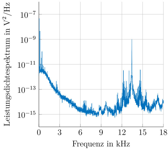
(a) Rauschspektrum
