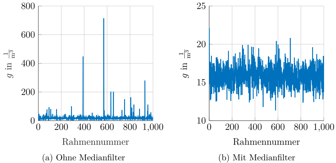
Abbildung 4.7: Auswertung des Distanzmerkmal anhand eines Laborsignals: In (a) ist der Verlauf des Distanzmerkmals ohne Medianfilter dargestellt, zum Vergleich dazu ist in (b) der Verlauf mit Medianfilter dargestellt. Die Rahmenlänge beträgt 512.
