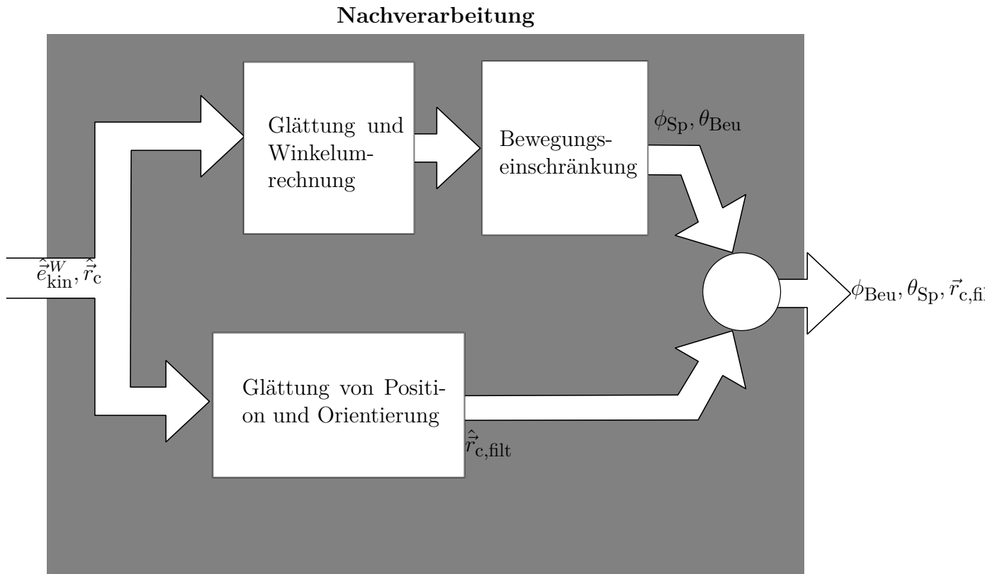
Abbildung 4.25: Übersicht des Nachverarbeitungsmodul: Auf der linken Seite sind die ungefilterten Schätzungen als Eingangsdaten dargestellt. Sowohl die absolute Position als auch die Orientierungen der kinematischen Elemente werden mit einem Tiefpass gefiltert. Die Orientierungen werden dann in Winkel umgerechnet und anhand bekannter Anatomie eingeschränkt. Die Ausgangsdaten sind dann die gefilterte Position, sowie die gefilterten Gelenkwinkel.
