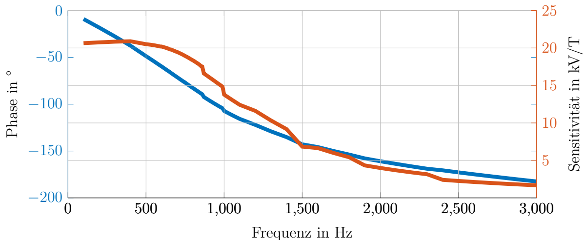
Abbildung 2.7: Verlauf von Sensitivität und Phase in Abhängigkeit der Frequenz
