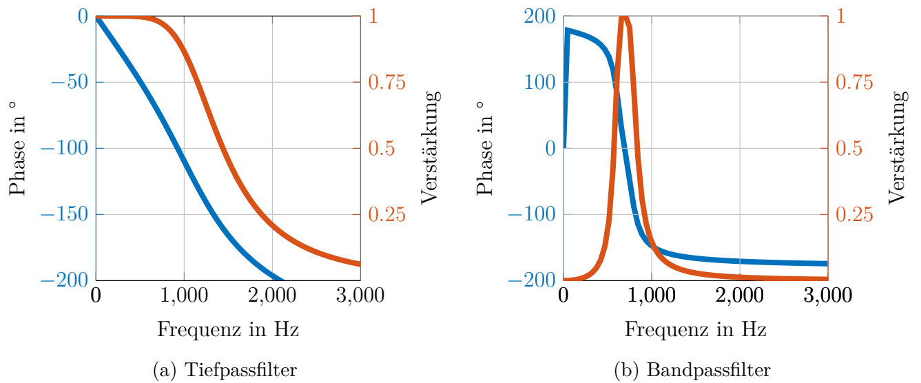
Abbildung 4.3: Vorverarbeitungsfilter: Auf der linken Seite ist der Tiefpassfilter zur Entzerrung des Stromsignals, auf der rechten Seite ist der Bandpassfilter zur Filterung von Störungen dargestellt.
