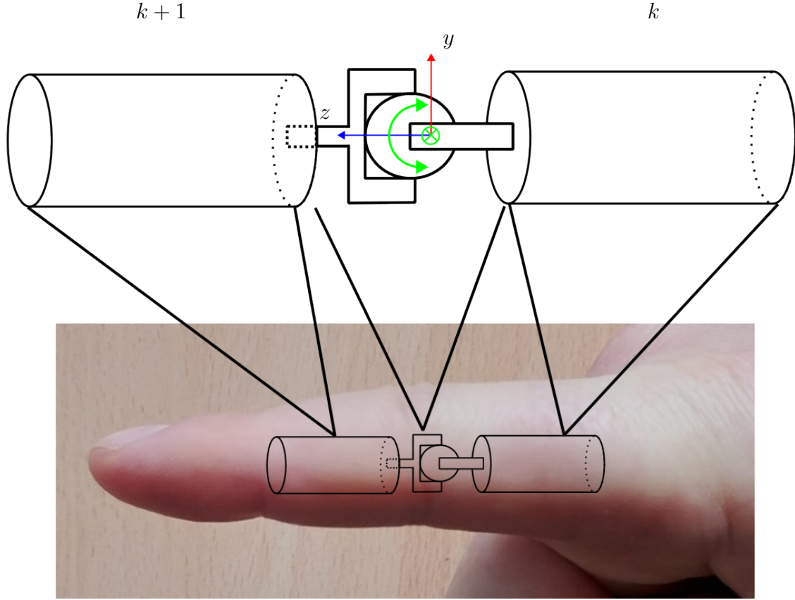
Abbildung 2.3: Modellierung einer kinematischen Kette: Die Abbildung zeigt eine kinematische Kette bestehend aus zwei Elementen mit dem zugehörigen Koordinatensystem. Unten ist exemplarisch ein Finger mit der zugehörigen Modellierung dargestellt.
