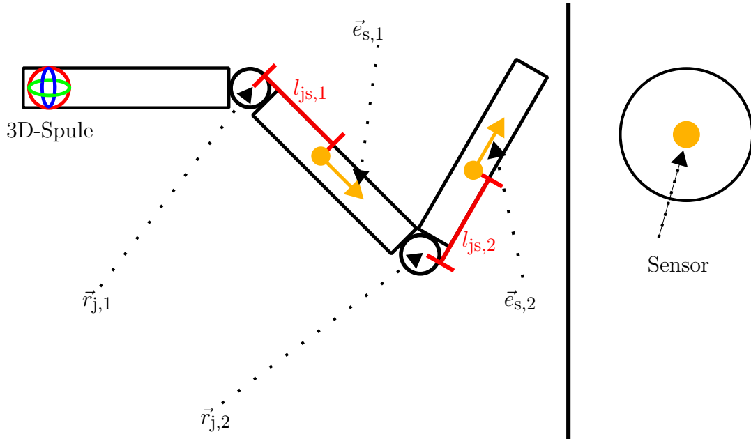
Abbildung 4.9: Sensor- und Quellenanordnung: Die kinematische Kette besteht aus zylinderförmigen Element, sowie Gelenke die diese verbinden und die Möglichkeit haben diese zu bewegen. Die linke Seite zeigt die Anordnung der Quellen und Sensoren auf der kinematischen Kette. Auf dem ersten Element ist eine 3D-Spule angebracht. Die weiteren Elemente sind mit Sensoren ausgerüstet. Diese sind auf der Mittelachse des kinematischen Elements, außerdem ist die sensitive Achse des Sensors mit der Symetrieachse des Elements ausgerichtet (siehe rechter Teil).
