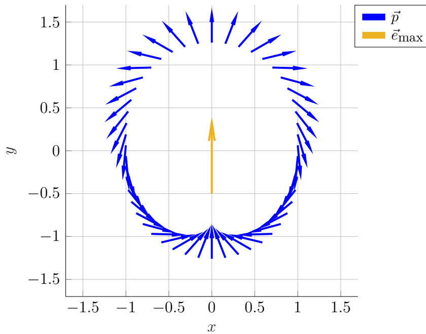
Abbildung 3.8: Potentielle Posen der Sensoren: In der Mitte ist ein MV in y -Richtung dargestellt. Die blauen Vektoren zeigen potentielle Posen, Positionen mit den zugehörigen Orientierungen. Der Anfang der Pfeile definiert die Position und die Richtung des Pfeils die zugehörige Orientierung.
