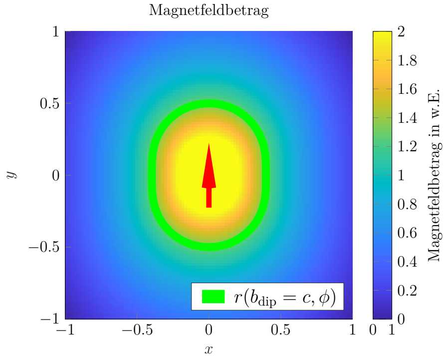
Abbildung 3.2: Die Abbildung zeigt exemplarisch den Verlauf des Magnetfeldbetrags. In der Mitte (roter Pfeil) ist ein magnetischer Dipol in y -Richtung polarisiert. Die grüne Kurve zeigt beispielhaft den Verlauf von r(b_{\text{Dip}} = c, \phi) .
