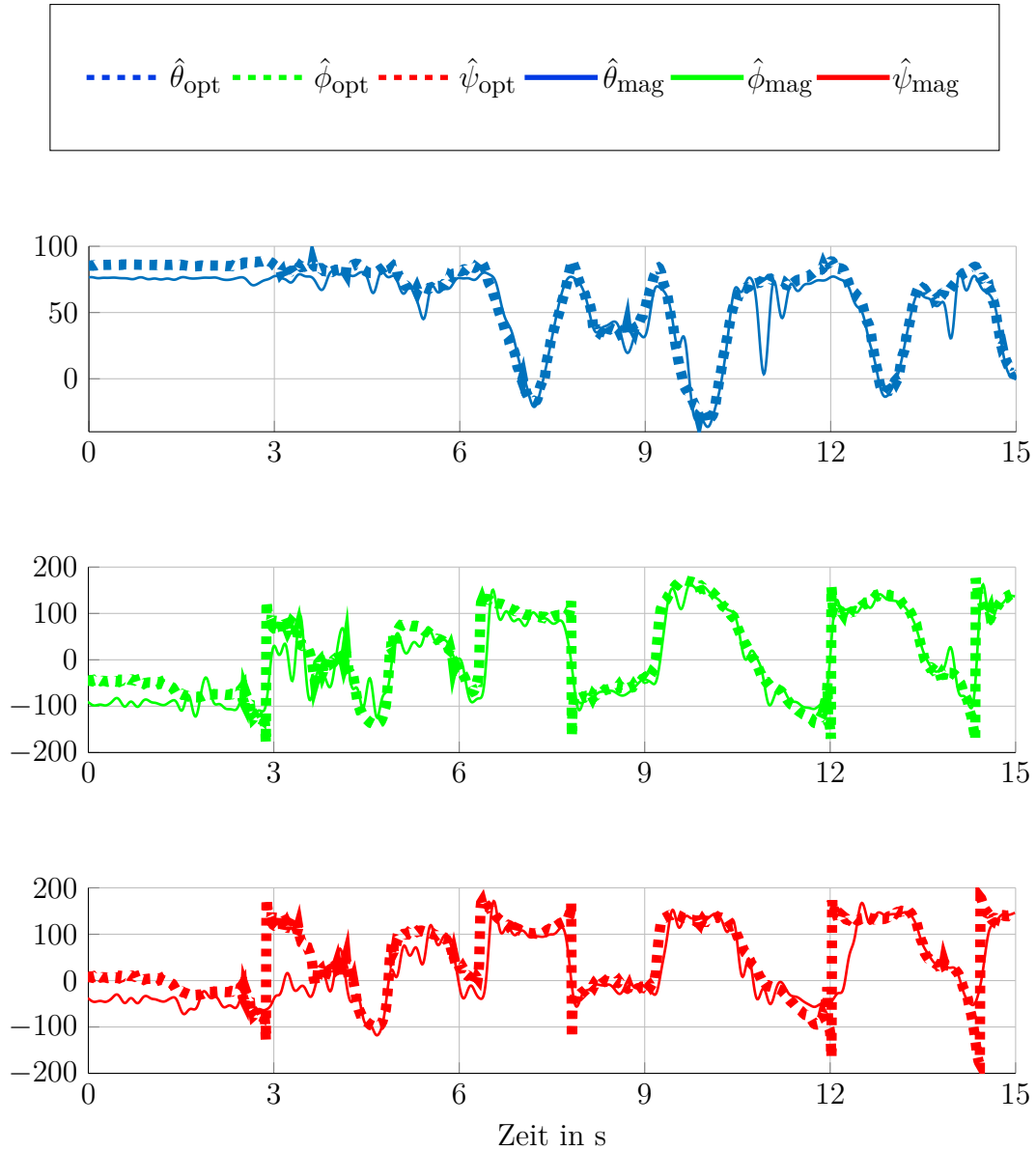
Abbildung 5.23: Ergebnis der dynamischen Evaluation der Orientierungsschätzung: Die optischen Schätzungen sind
