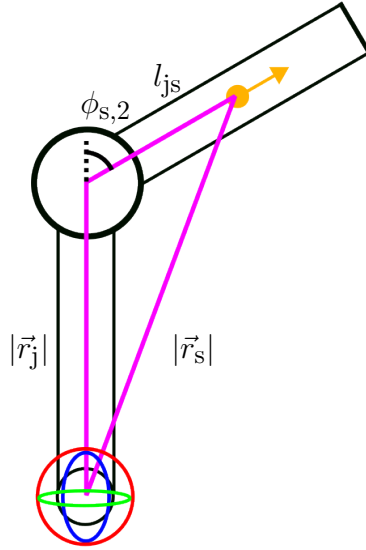
Abbildung 4.22: Distanz zu Winkel: Die Abbildung zeigt eine kinematische Kette mit zwei Elementen. Auf dem ersten Element (unten) ist ein Akktuator angebracht, auf dem zweiten ein Sensor(orange). In pink ist ein Dreieck eingezeichnet mit den zugehörigen Längen.
