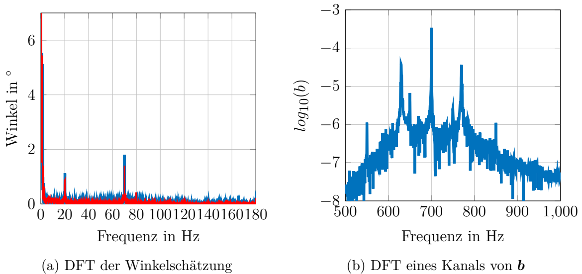
Abbildung 5.16: Frequenzanalyse der Winkelschätzung und der magnetischen Eingangssignale, es ist jeweils das Signal des ersten Elements dargestellt.
