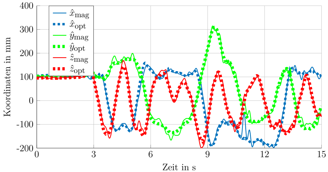
Abbildung 5.22: Ergebnis der dynamischen Evaluierung der Positionsschätzung: Es sind die drei Positionskomponenten dargestellt. Die magnetischen Schätzungen sind in durchgezogenen Linien und die optischen in gestrichelten Linien dargestellt.
