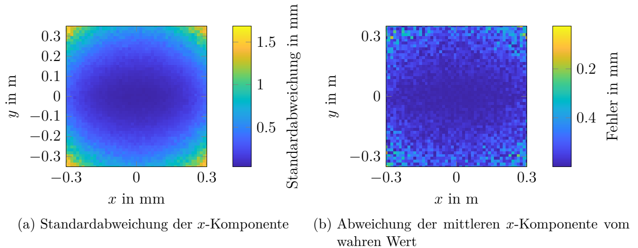
Abbildung 5.18: Ergebnisse der Simulation zur Überprüfung der Robustheit der Positionsschätzung unter Einfluss von weißem Rauschen
