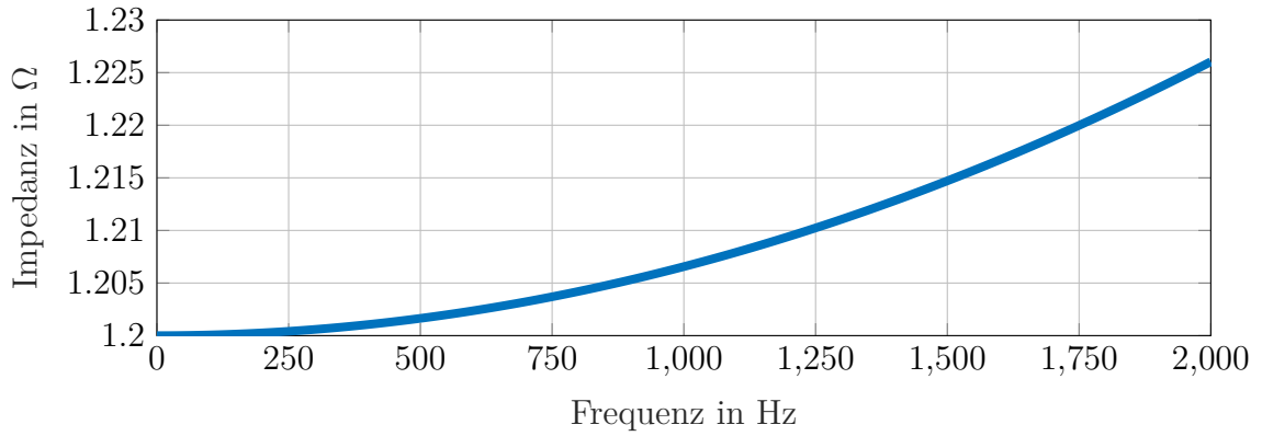
Abbildung 3.5: Frequenzabhängiger Impedanzverlauf einer der Spulen
