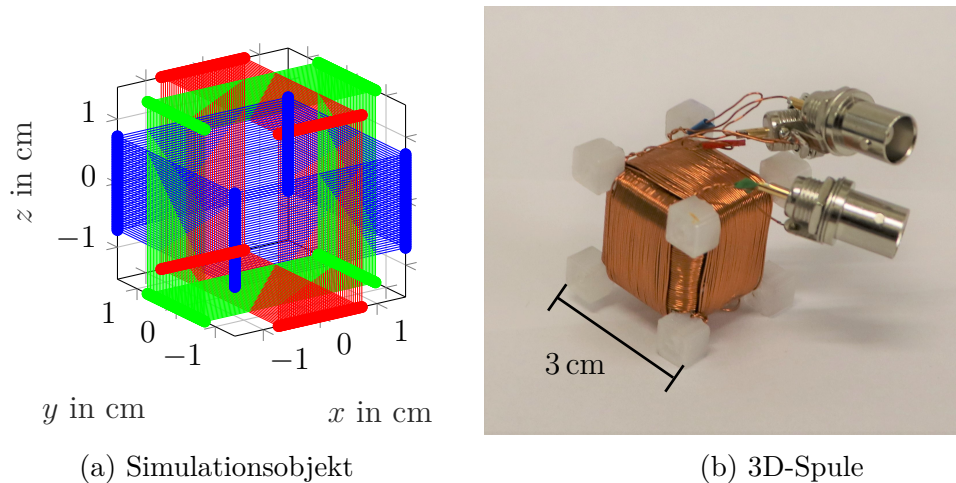
Abbildung 3.4: 3D-Spule: (a) skizziert das modellierte Simulationsobjekt, wobei rot für die x -Spule, grün für die y -Spule und blau für die z -Spule steht. Ein Foto der entsprechenden Realisierung ist in (b) zu sehen.
