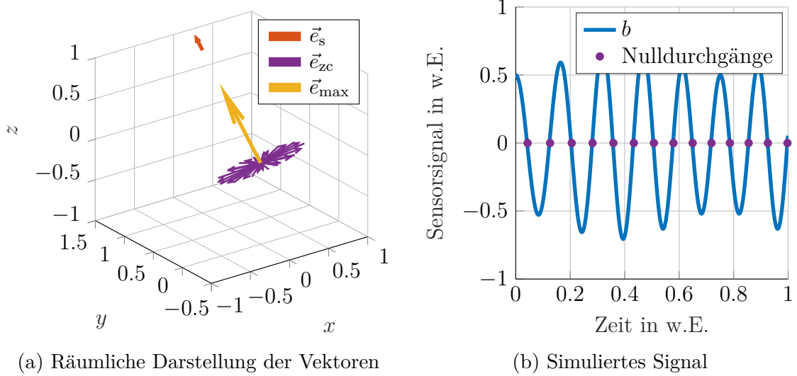
Abbildung 4.6: Die linke Abbildung zeigt beispielhaft einen MV im Ursprung (gelb), die Position und Orientierung (orange) des Sensors und die entsprechende Ebene der Nulldurchgangsvektoren (lila). Auf der rechten Seite ist b(n) als Funktion der Zeit dargestellt. Die Zeiten, in denen ein Nulldurchgang erreicht wird, sind mit einem lila Punkt markiert. Die Simulation arbeitet mit einer Quelle, die mit N_\omega = \omega_\theta / \omega_\phi = 10 angesteuert wird. Die absoluten Werte/Längen sind nicht relevant, da zum einen das relative Verhältnis zwischen den Vektoren und zum anderen die Nulldurchgänge von Interesse sind.
