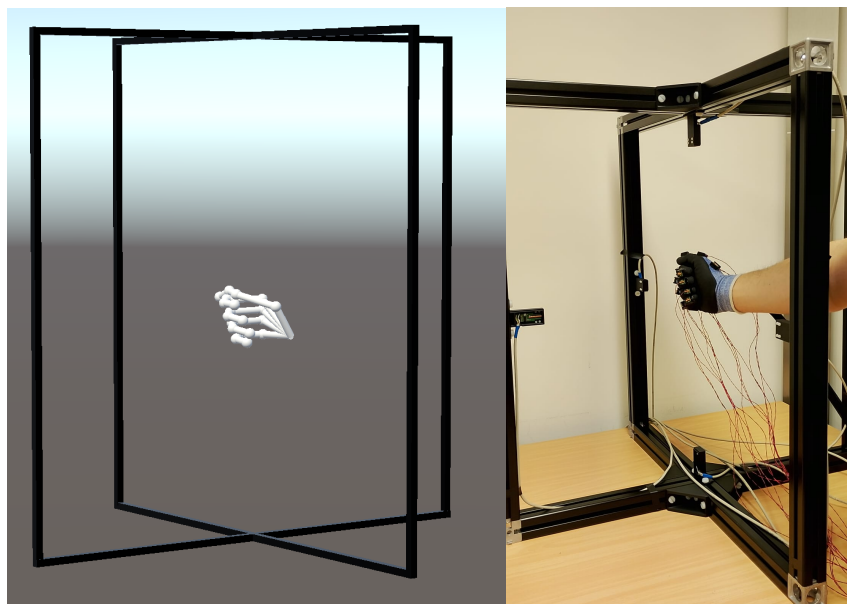
Abbildung 6.3: Die linke Seite zeigt die Visualisierung der Schätzung, auf der rechten Seite ist die zugehörige Hand mit Prototyp zu sehen.
