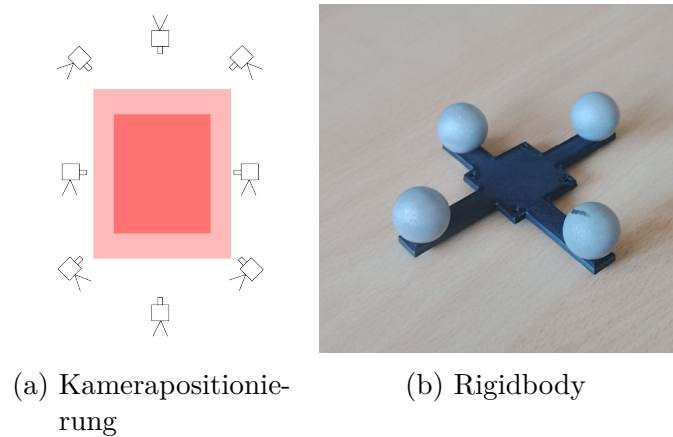
Abbildung 2.5: Aufbau OMC: a zeigt eine mögliche Kameraanordnung. In Dunkelrot ist dabei der Bereich zu sehen, der von allen acht Kameras eingesehen wird. Der hellrote Bereich wird dann nur von einem Teil der Kameras erreicht. In b ist beispielhaft ein Rigidbody dargestellt. Dieser besteht aus einem 3D-Druckteil an dem insgesamt 4 optische Marker angebracht sind.
