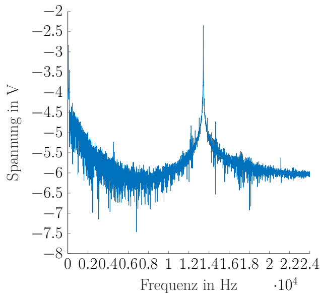
(a) Rauschspektrum
