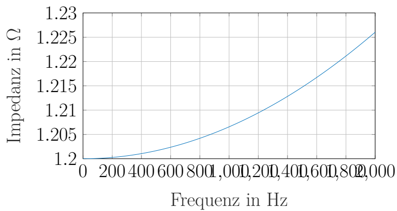
Abbildung 3.5: Frequenzabhängiger Impedanzverlauf der 3D-Spule
