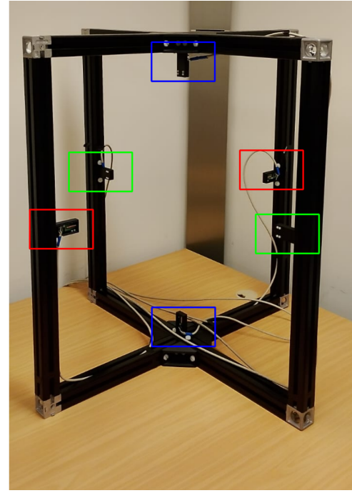
(b) Laboraufbau
