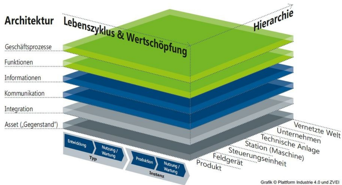
Abbildung 3: RAMI 4.0: Referenzarchitekturmodell Industrie 4.0 als dreidimensionales Schichtenmodell mit den Achsen „Life Cycle & Value Stream“, „Hierarchy Levels“ und „Layers“ (Quelle: DIN SPEC 91345 [12]).
