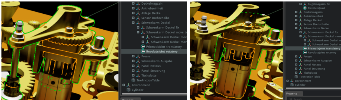
Abbildung 6: Verschachtelte Gelenke am Schwenkarm-Deckel: RevoluteJoint rotatory (links) und PrismaticJoint translatory (rechts) mit Kollisionskonturen (grün).
