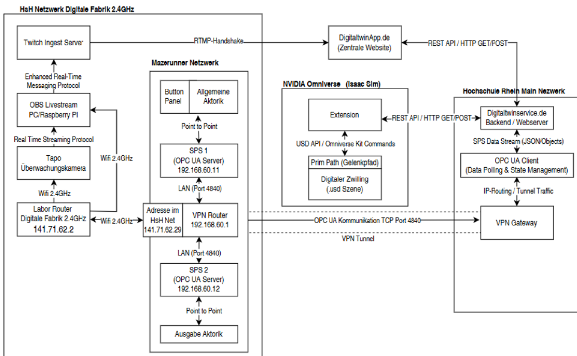
Abbildung 7: Systemarchitektur des Maze-Runner-Digitalen-Zwillings: SPS-Netzwerk (links), Omniverse-Extension (Mitte) und DigitalTwinService mit VPN-Gateway (rechts).
