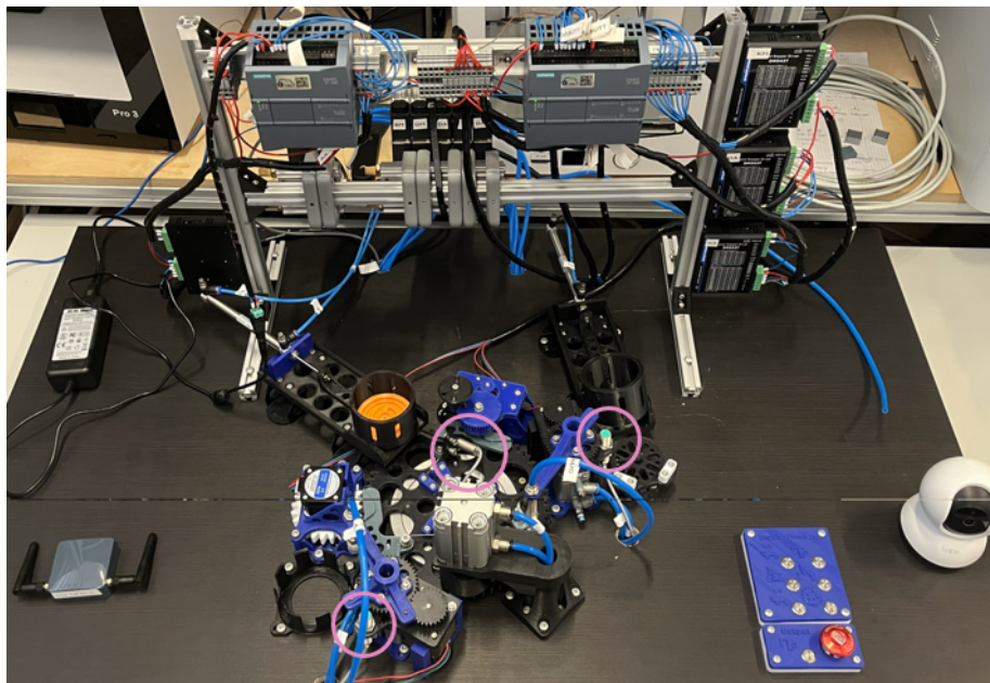
Abbildung 8: IST-Zustand der Maze-Runner-Anlage im Hochschullabor (Aufnahme von oben).
