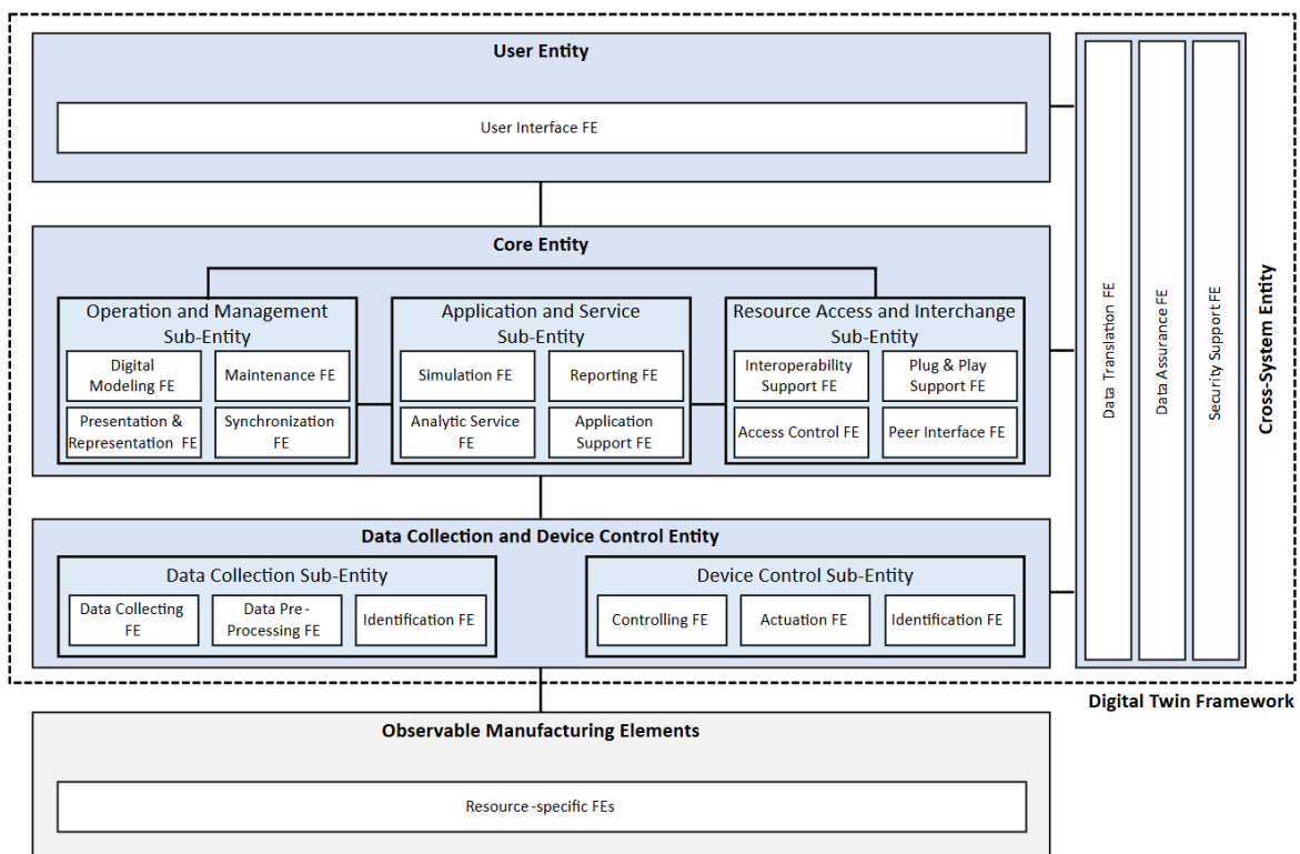
Abbildung 4: Digital Twin Framework nach ISO 23247: Struktur aus User Entity, Core Entity, Data Collection and Device Control Entity sowie Cross-System Entity mit den jeweiligen funktionalen Elementen (FE) (Quelle: [13]).
