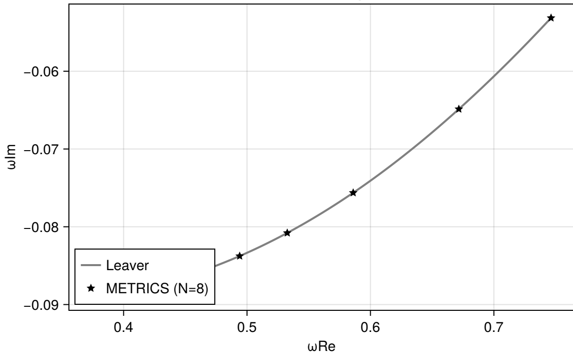
022-mode QNM frequencies
