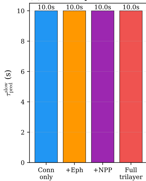
(d) Slow-component horizon
