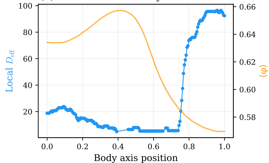
(d) Local dimensionality vs coherence
