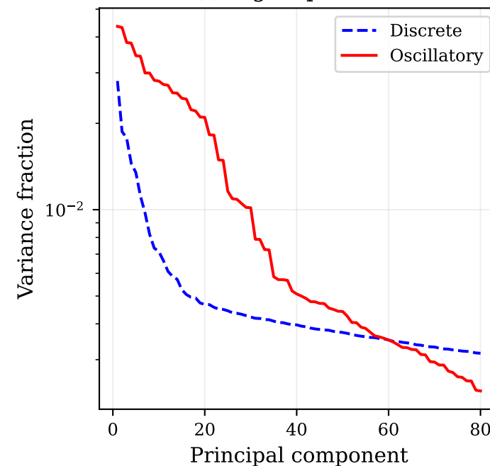
(f) Eigenspectrum
