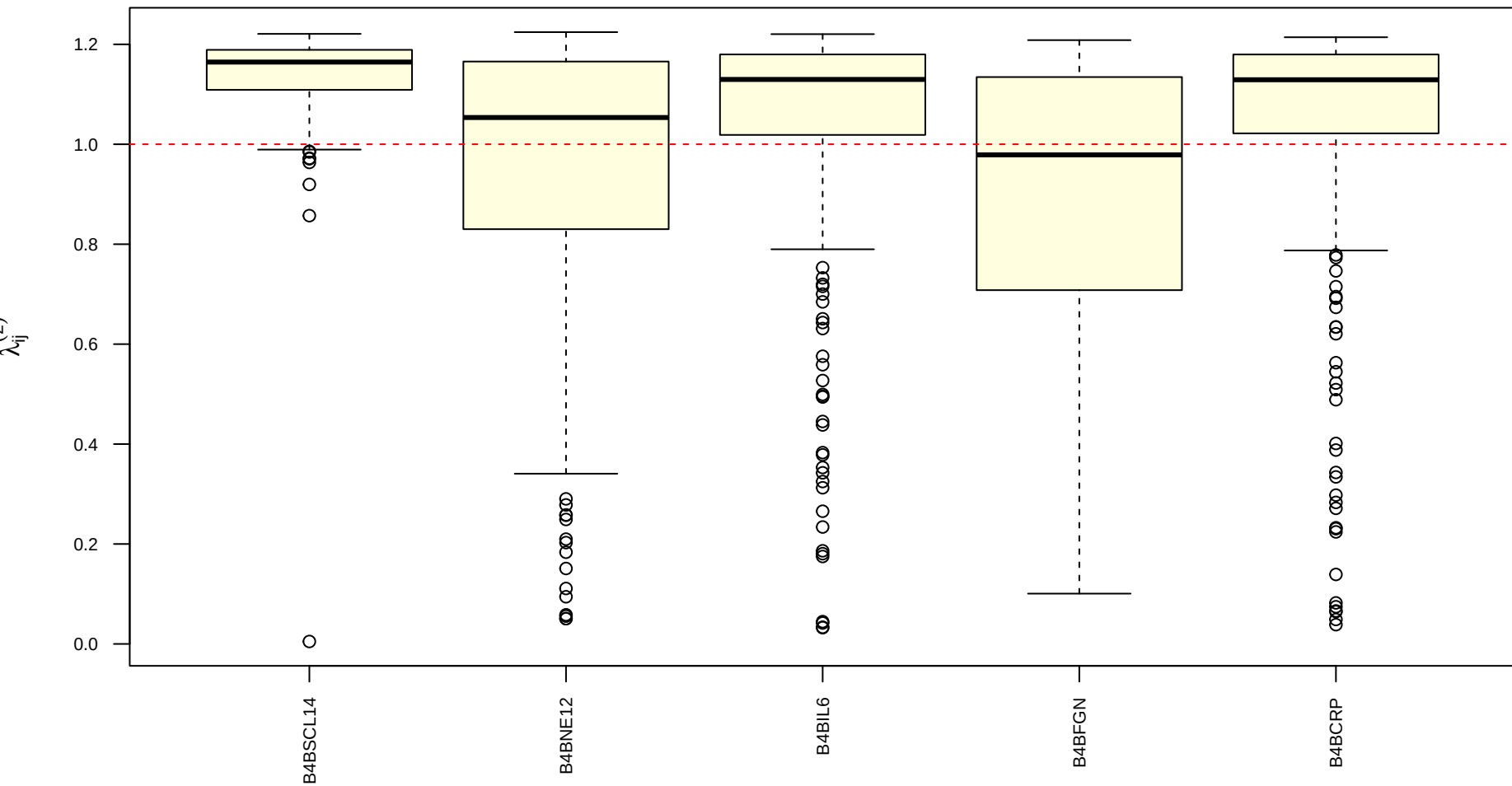
Posterior Mean \lambda_{ij}^{(2)} by Item
