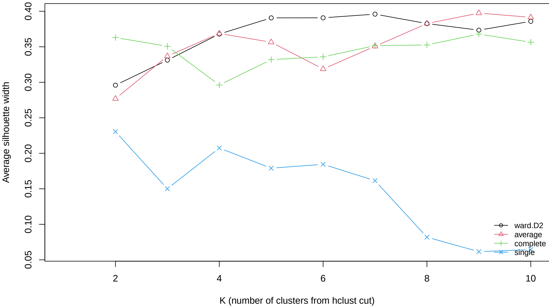
Silhouette vs K per linkage
