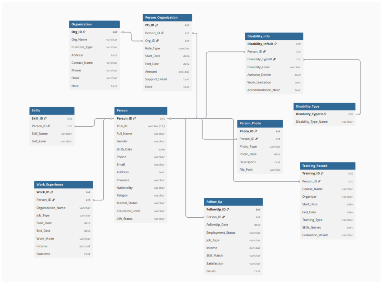
ER-Diagram ระบบฐานข้อมูลคนพิการ โครงการฝึกอบรม-ฝึกงานคนพิการฯ มจร.
