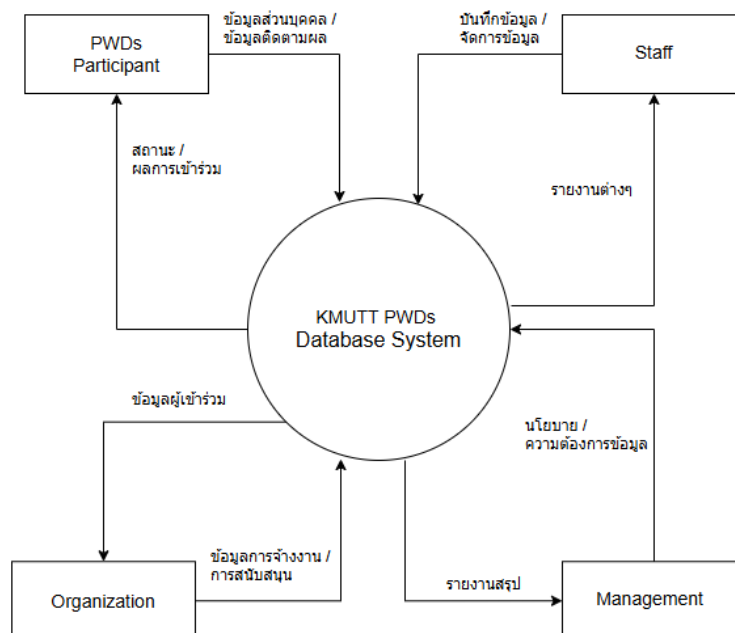
แผนภาพเชิงระบบ Data Flow Diagram Level 0
