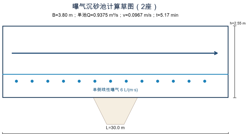
图 6-1 曝气沉砂池计算草图
