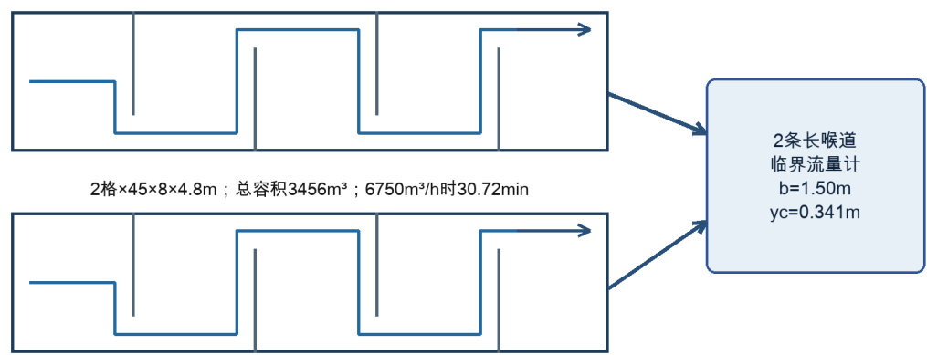
接触消毒与计量终端计算草图
