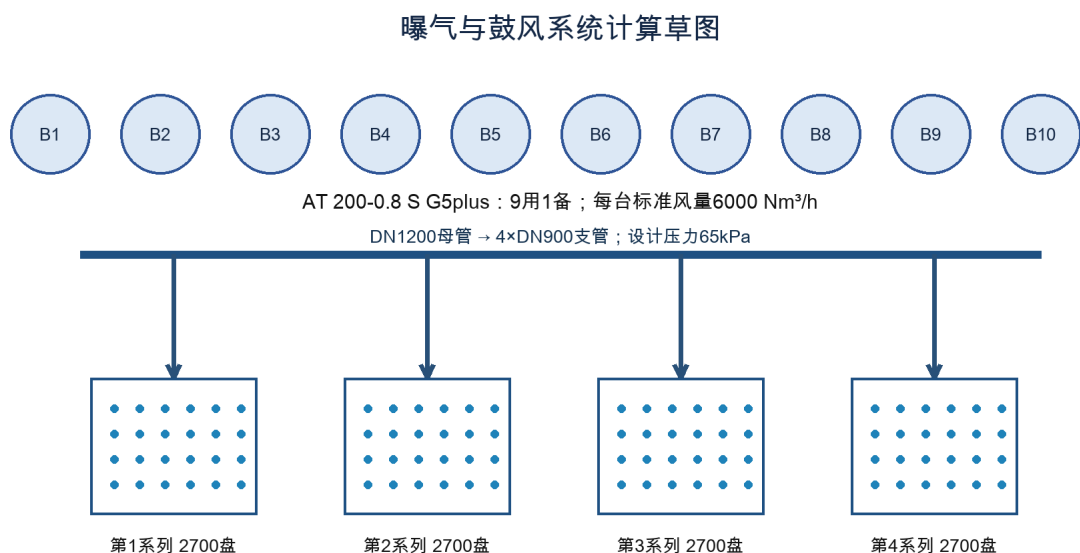
图 10-1 曝气与鼓风系统计算草图
