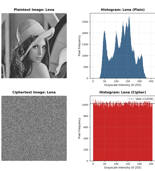
(a) Lena: Ảnh gốc, ảnh mã hóa nhiễu trắng và biểu đồ histogram.
