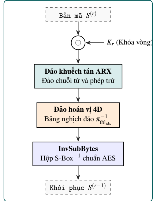
Hình 1: Kiến trúc tổng thể của Rubik-4D: (a) Luồng mã hóa gồm SubBytes, hoán vị siêu lập phương SO(4) , khuếch tán ARX 32-bit và AddRoundKey; (b) Luồng giải mã sinh ảnh nghịch đảo tương ứng.
