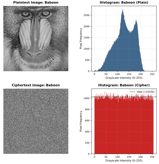
(b) Baboon: Ảnh gốc, ảnh mã hóa nhiễu trắng và biểu đồ histogram.
