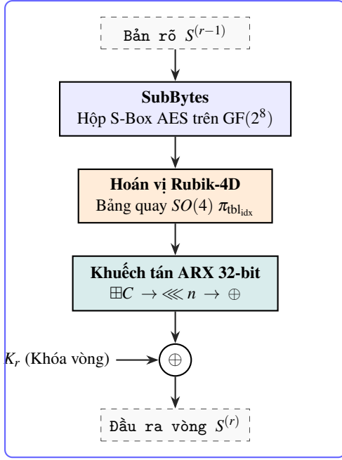
Hình 1: Kiến trúc tổng thể của Rubik-4D: (a) Luồng mã hóa gồm SubBytes, hoán vị siêu lập phương SO(4) , khuếch tán ARX 32-bit và AddRoundKey; (b) Luồng giải mã sinh ảnh nghịch đảo tương ứng.
