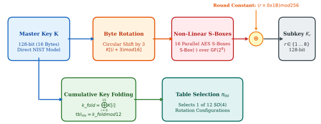
Hình 3: Quy trình sinh khóa vòng của Rubik-4D: (1) Nạp trực tiếp khóa chính 128-bit theo chuẩn NIST FIPS 197; (2) Gập khóa k\_fold chọn bảng hoán vị SO(4) \pi_{tbl_{idx}} ; (3) Sinh khóa con đệ quy qua các vòng r = 1 \dots 8 kết hợp phép dịch vòng byte, 16 hộp S-box AES song song và hằng số vòng ( r \times 0x1B ).
