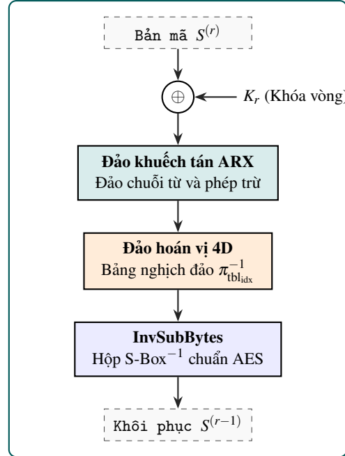
Hình 2: Kiến trúc tổng thể của Rubik-4D: (a) Luồng mã hóa gồm SubBytes, hoán vị siêu lập phương SO(4) , khuếch tán ARX 32-bit và AddRoundKey; (b) Luồng giải mã sinh ảnh nghịch đảo tương ứng.
