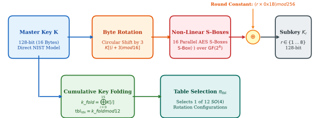
Hình 3: Quy trình sinh khóa vòng của Rubik-4D: (1) Nạp trực tiếp khóa chính 128-bit theo chuẩn NIST FIPS 197; (2) Gập khóa k\_fold chọn bảng hoán vị SO(4) \pi_{\text{tbl\_idx}} ; (3) Sinh khóa con đệ quy qua các vòng r = 1 \dots 8 kết hợp phép dịch vòng byte, 16 hộp S-box AES song song và hằng số vòng (r \times 0x1B) .
