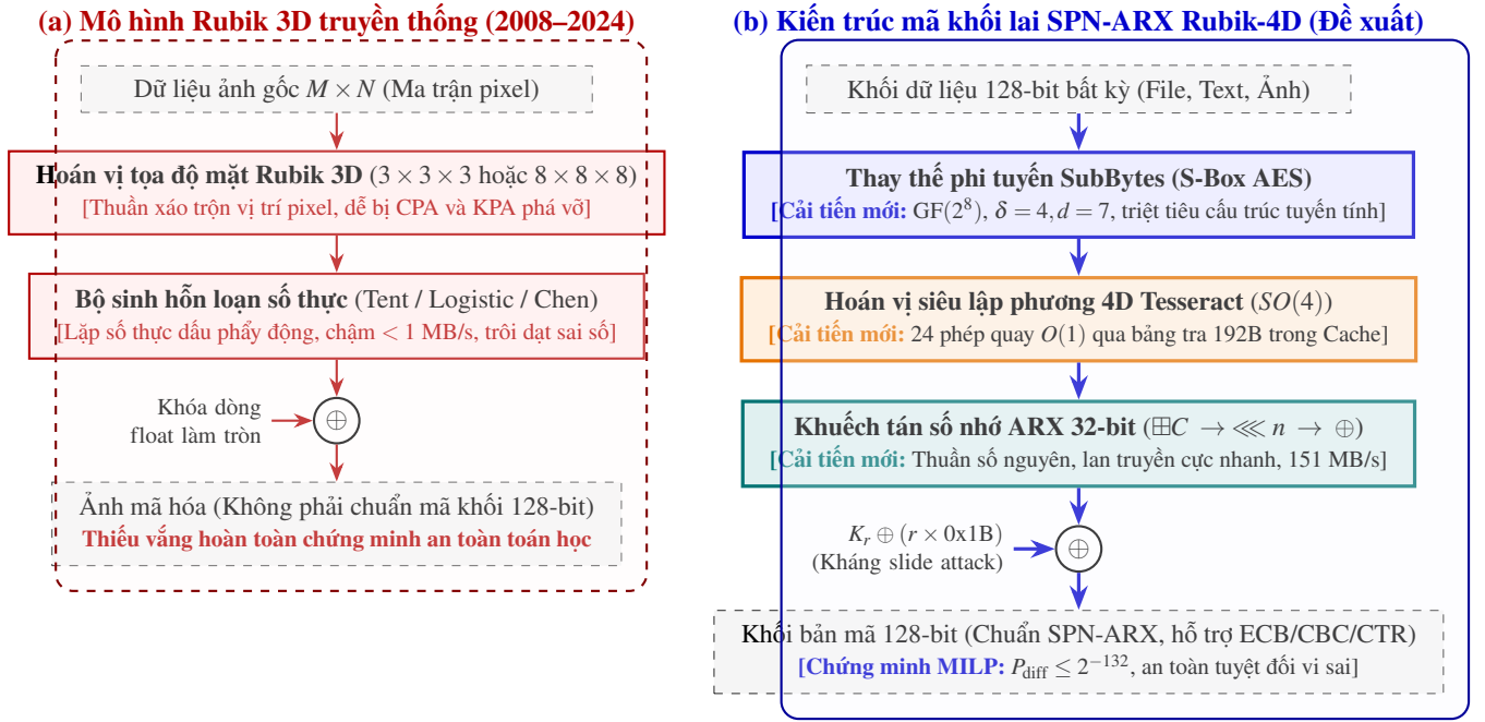
Hình 1: Sơ đồ đối sánh kiến trúc: (a) Mô hình Rubik 3D truyền thống (xáo trộn tọa độ điểm ảnh kết hợp hỗn loạn số thực, chậm và thiếu chứng minh toán học); (b) Kiến trúc mã khối Rubik-4D đề xuất với các khối cải tiến đột phá (S-box AES phi tuyến, hoán vị siêu lập phương 4D SO(4) tra bảng O(1) , khuếch tán ARX 32-bit thuần số nguyên và chứng minh an toàn tự động bằng MILP).
