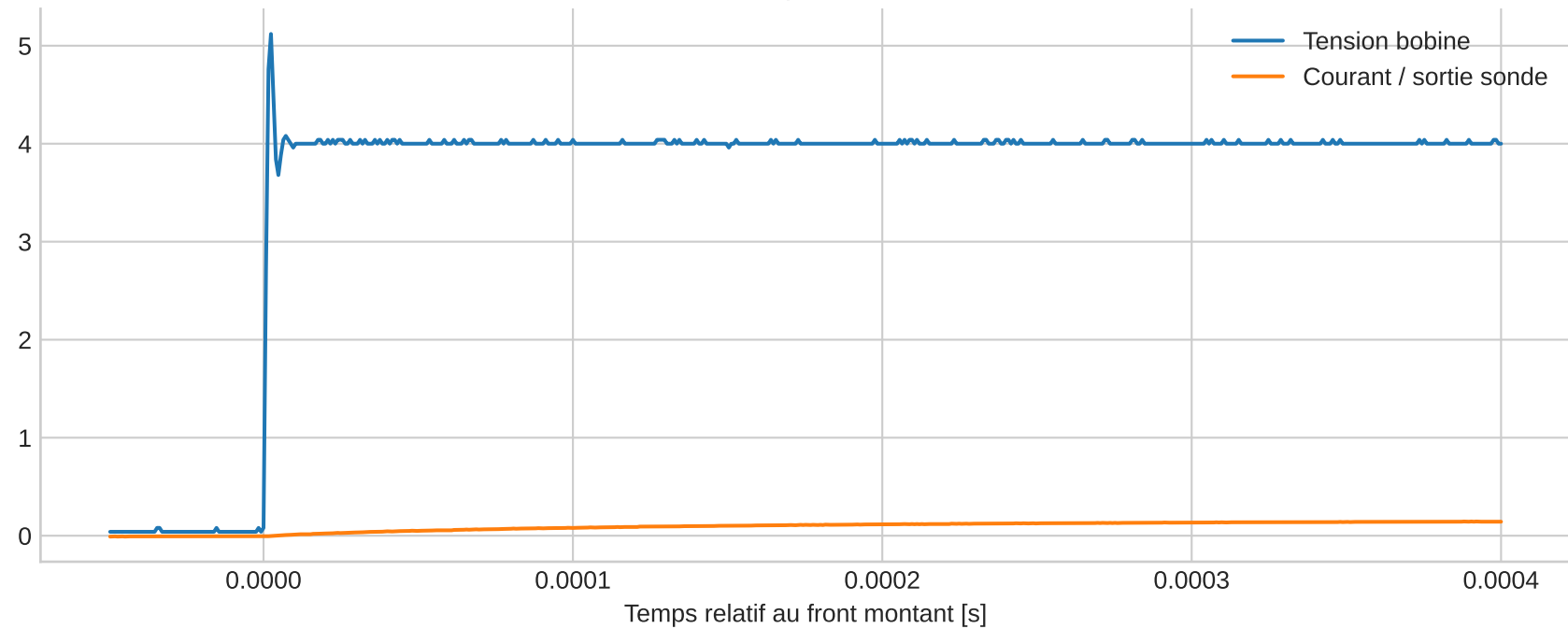
EX1 - Zoom sur la reponse avec mouvement
