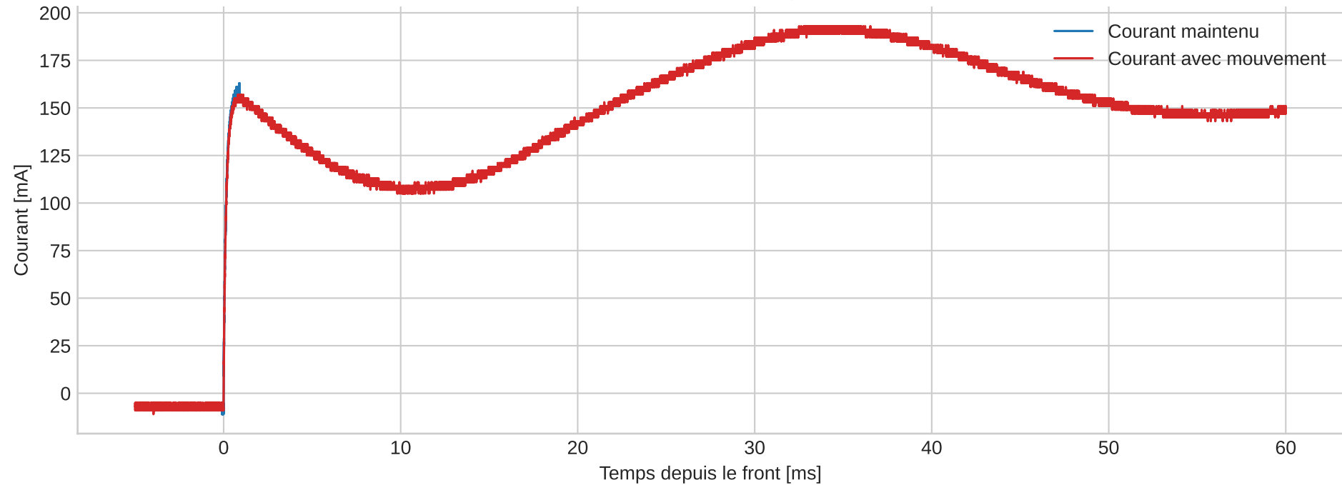
EX1 : effet de la f.c.e.m. sur la reponse en courant
