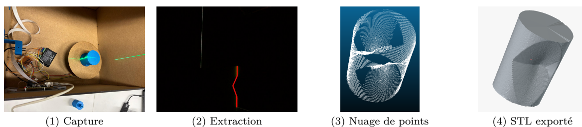
FIGURE 6 – Chaîne de traitement observée sur le prototype réel : de la capture image jusqu'au fichier STL.
